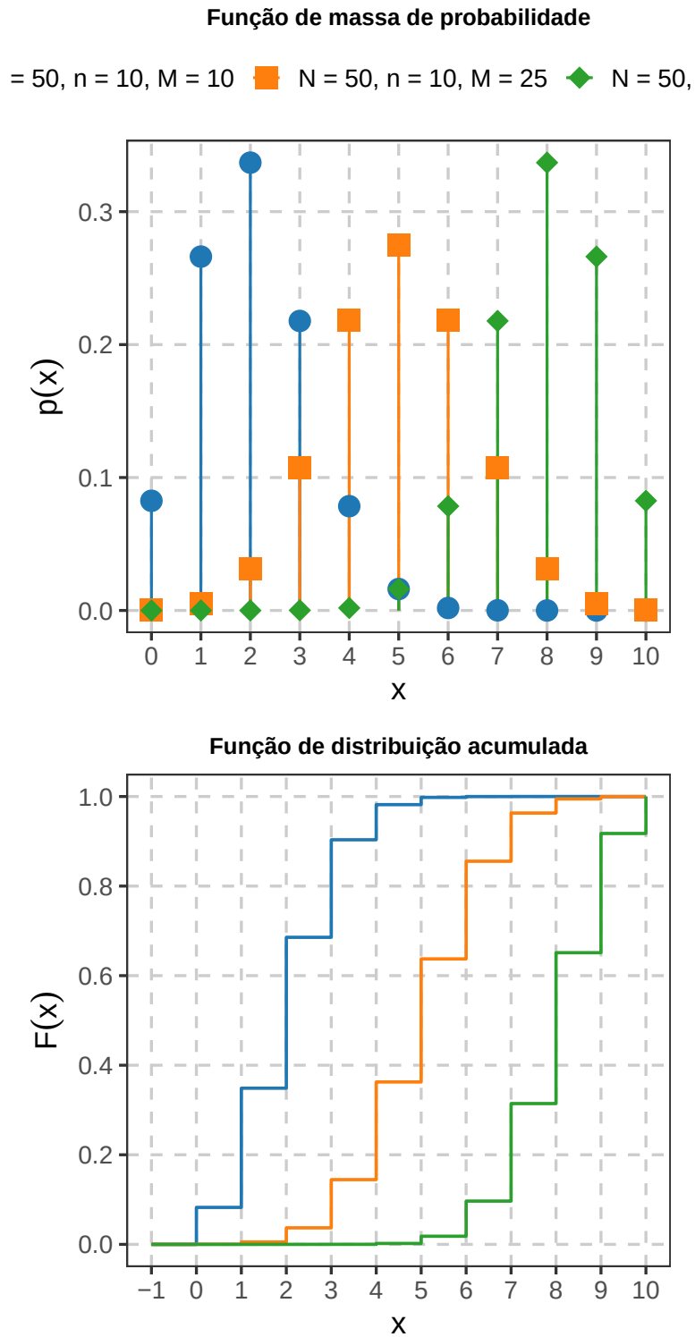
Figura 4: Função de massa de probabilidade e função de distribuição acumulada da distribuição hipergeométrica para diferentes parâmetros.
