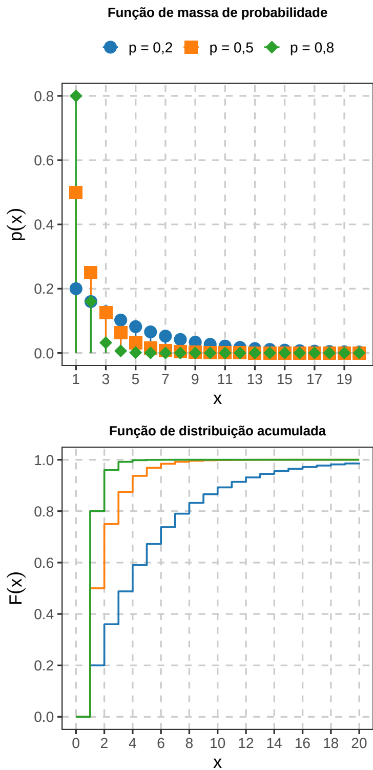
Figura 5: Função de massa de probabilidade e função de distribuição acumulada da distribuição geométrica para diferentes parâmetros.
