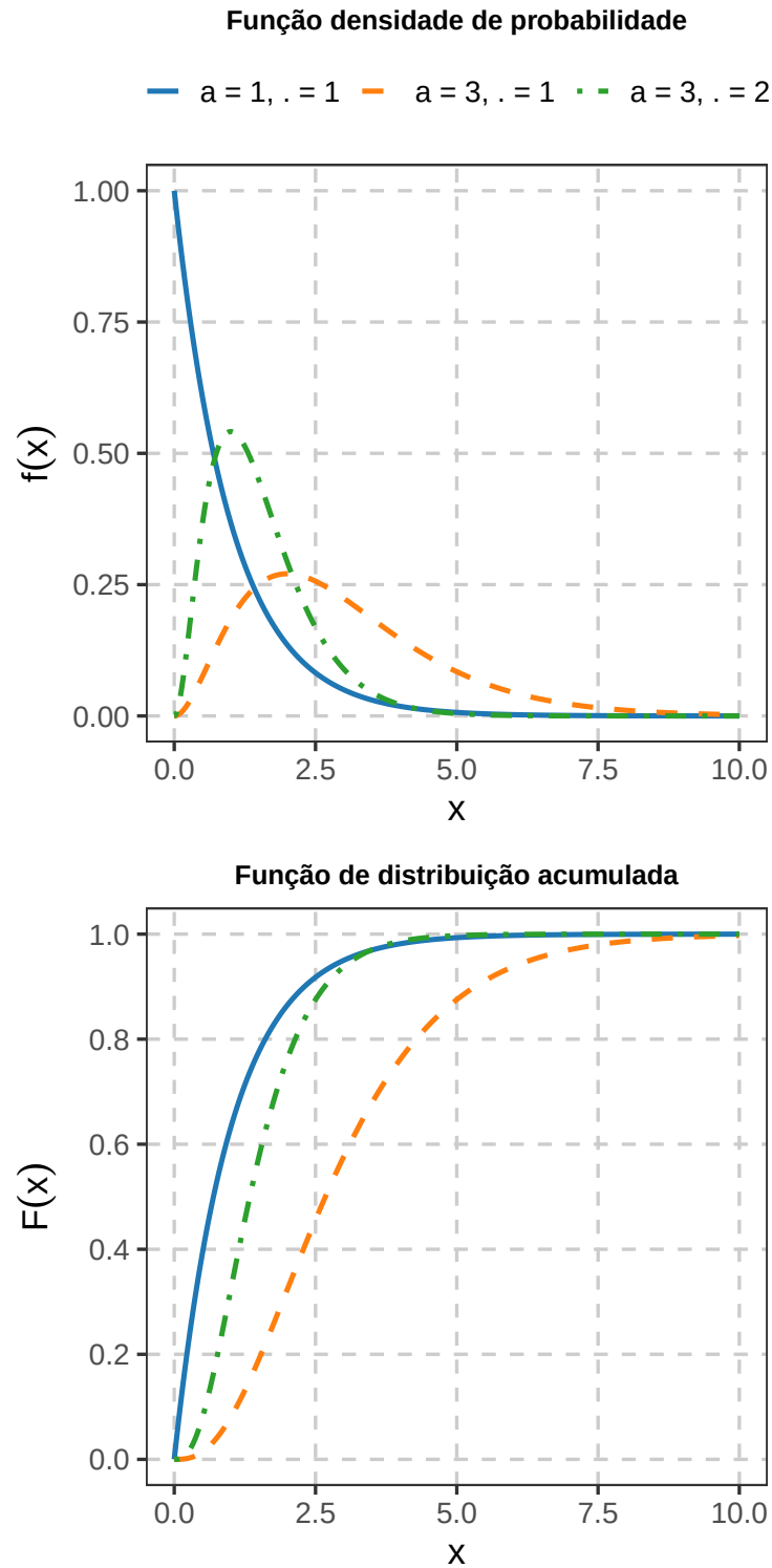
Figura 11: Função densidade de probabilidade e função de distribuição acumulada da distribuição gama para diferentes parâmetros.
