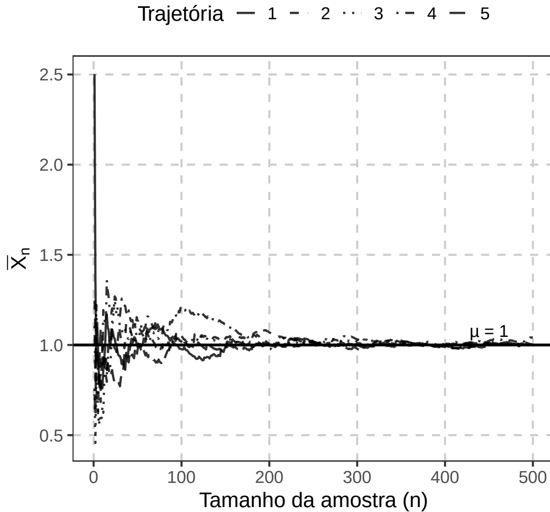
Figura 16: Trajetórias de médias acumuladas de amostras exponenciais com média \mu=1 . As médias amostrais tendem a se estabilizar em torno da média populacional à medida que n aumenta.
