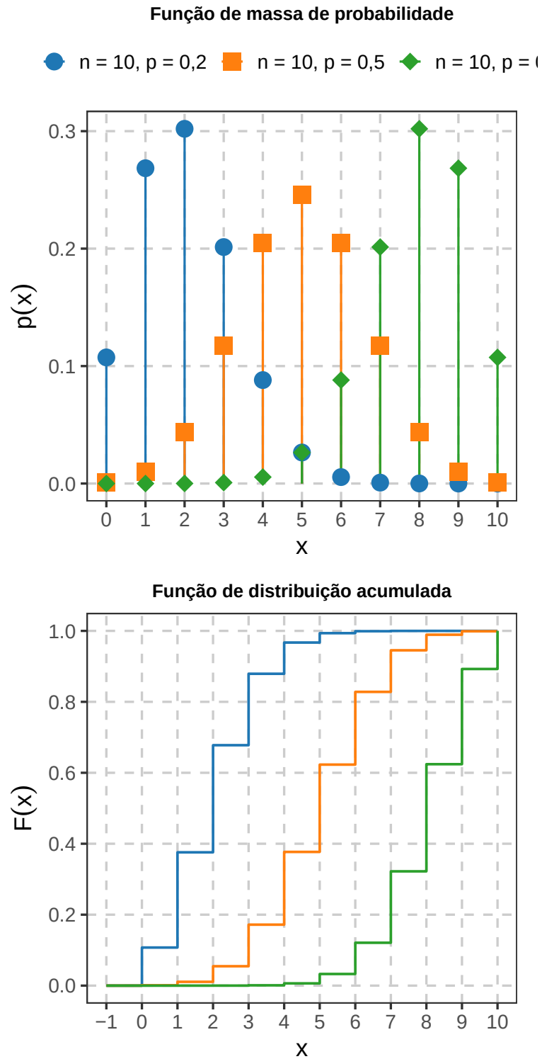
Figura 3: Função de massa de probabilidade e função de distribuição acumulada da distribuição binomial para diferentes parâmetros.
