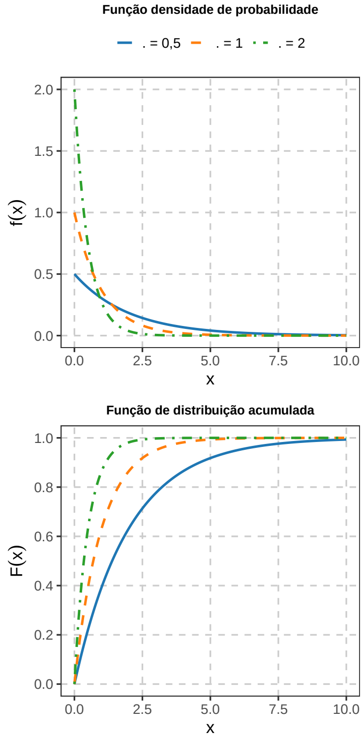
Figura 10: Função densidade de probabilidade e função de distribuição acumulada da distribuição exponencial para diferentes parâmetros.
