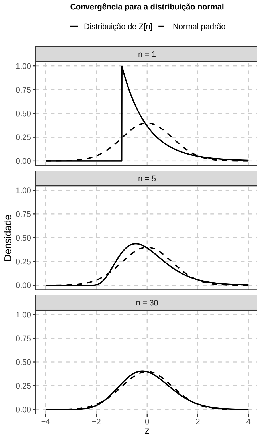
Figura 17: Densidade da média exponencial padronizada para diferentes tamanhos de amostra e densidade da distribuição normal padrão.
