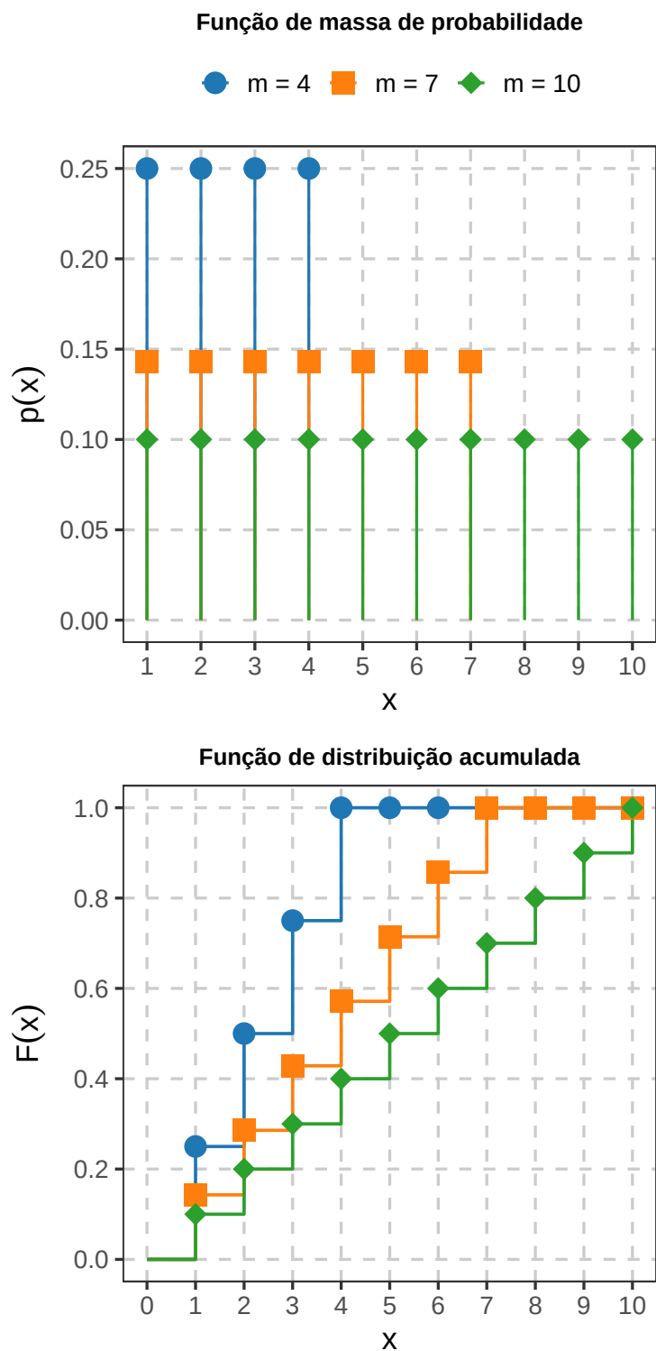
Figura 1: Função de massa de probabilidade e função de distribuição acumulada da distribuição uniforme discreta para diferentes parâmetros.
