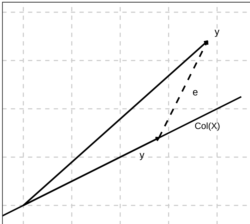
Figura 15: Representação geométrica de uma projeção ortogonal: o vetor y é decomposto na projeção y sobre um subespaço e no resíduo ortogonal e .
