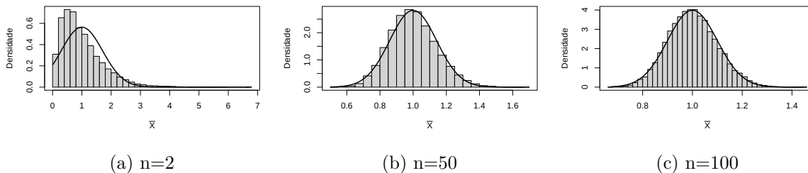
Figura 2.1: Distribuições simuladas da média de amostras exponenciais.
