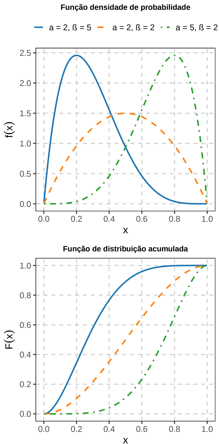
Figura 13: Função densidade de probabilidade e função de distribuição acumulada da distribuição beta para diferentes parâmetros.
