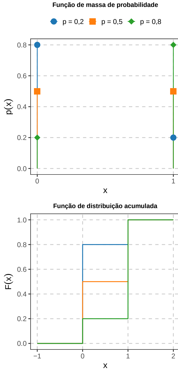
Figura 2: Função de massa de probabilidade e função de distribuição acumulada da distribuição de Bernoulli para diferentes parâmetros.
