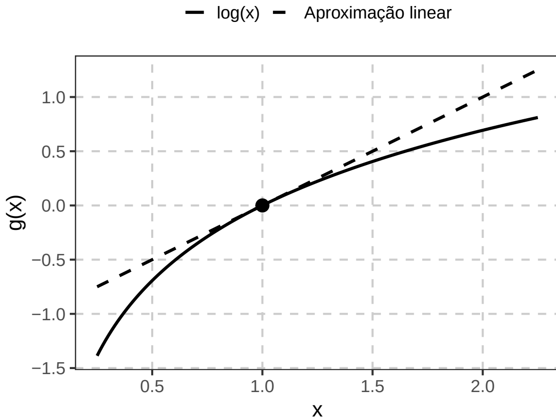
Figura 14: Função logarítmica e sua aproximação de Taylor de primeira ordem em torno de a=1 .
