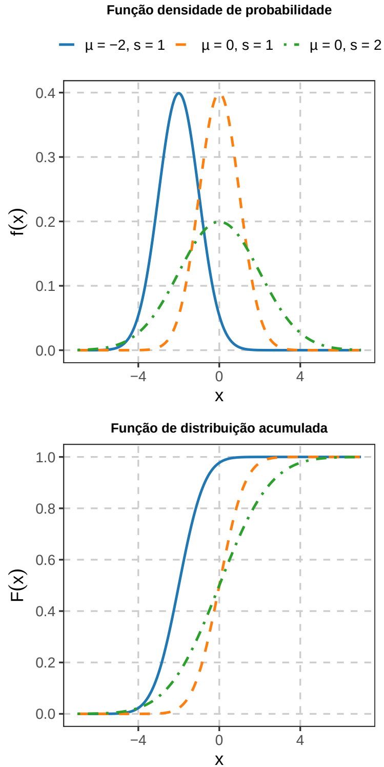
Figura 12: Função densidade de probabilidade e função de distribuição acumulada da distribuição normal para diferentes parâmetros.
