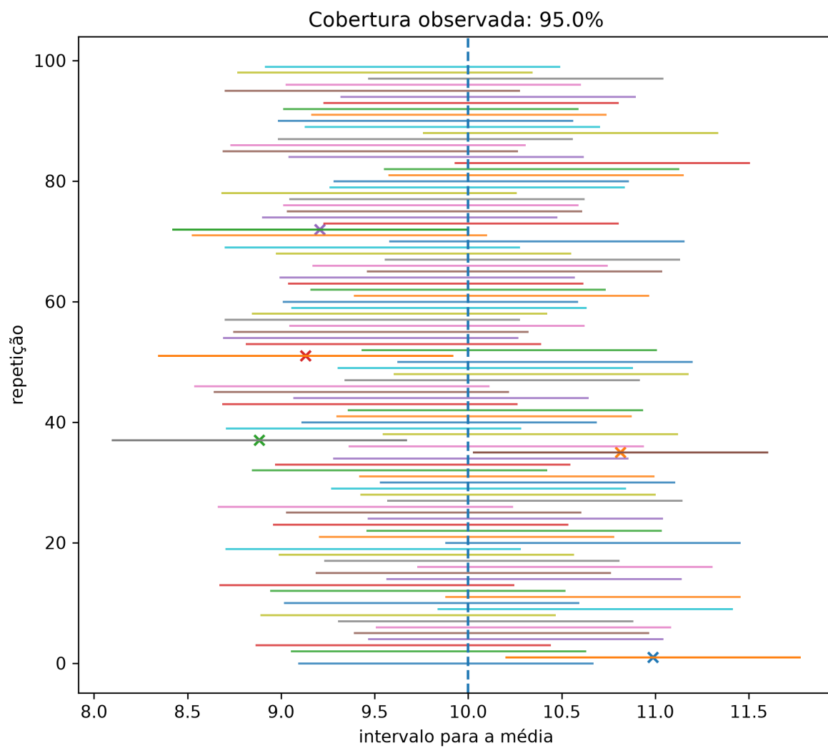
Figura 6.2: Simulação de intervalos de 95% para uma média normal.
