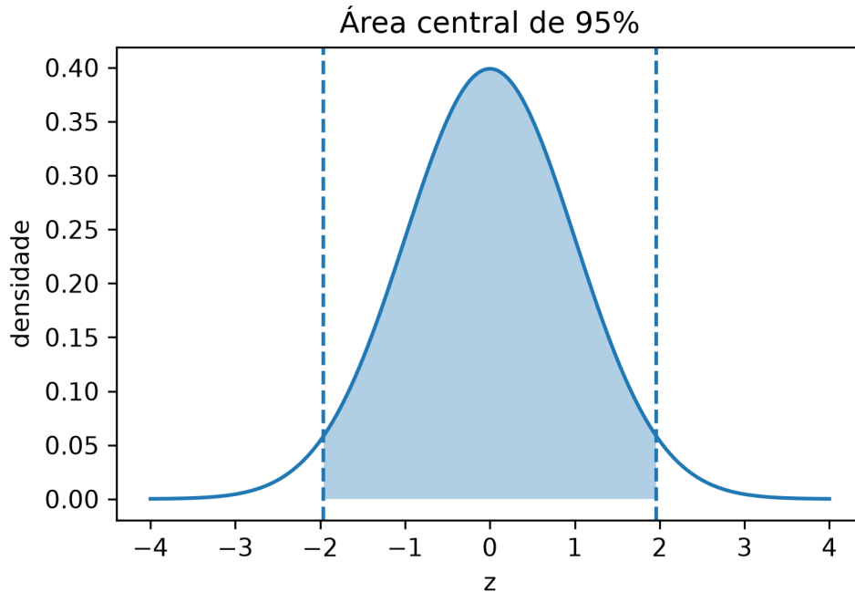
Figura 6.1: Região central de 95% da distribuição normal padrão.
