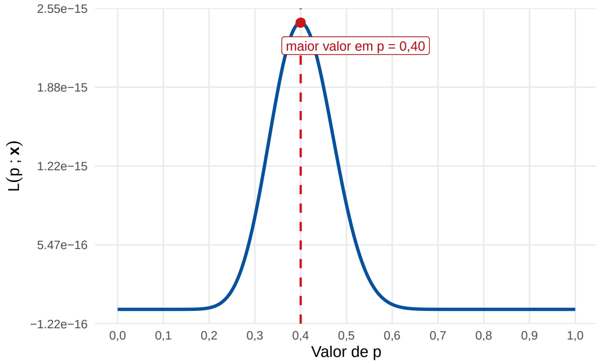
Figura 3.1: Função de verossimilhança para o modelo Bernoulli com n = 50 e v = 20 .
