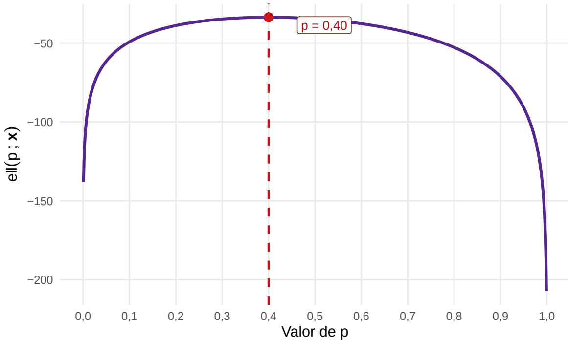
Figura 3.2: Função de log-verossimilhança para o modelo Bernoulli com n = 50 e v = 20 .
