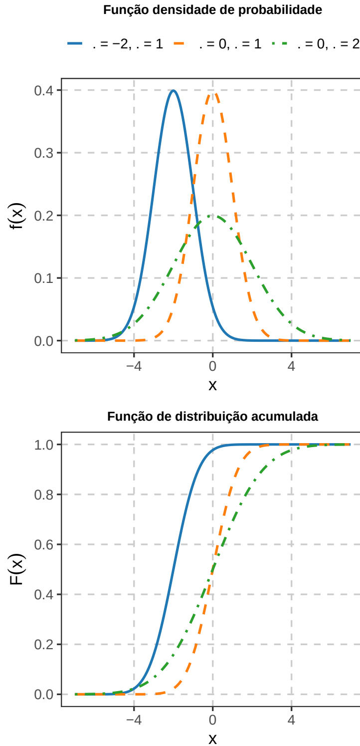
Figura 1.12: Função densidade de probabilidade e função de distribuição acumulada da distribuição normal para diferentes parâmetros.
