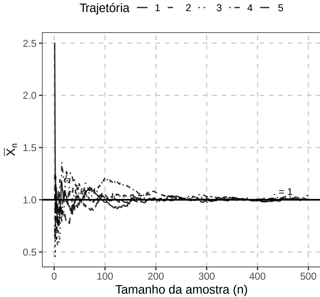
Figura 2.3: Trajetórias de médias acumuladas de amostras exponenciais com média 1.
