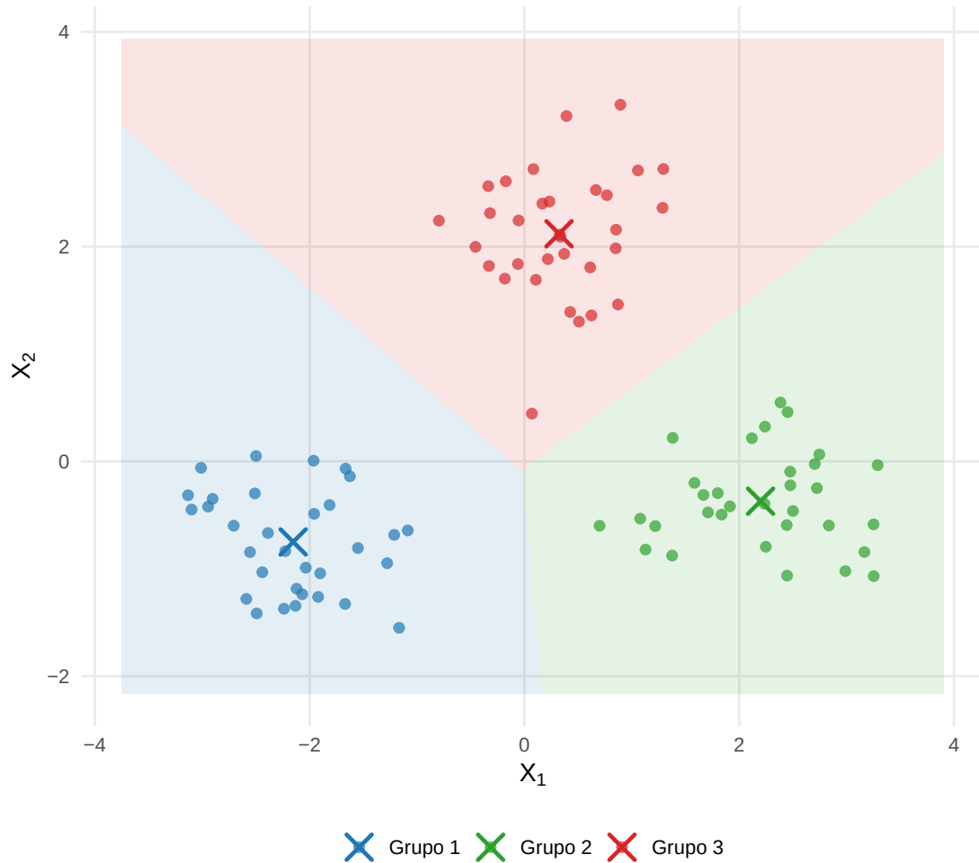
Figura 16.3: Centroides e regiões de alocação definidas pela distância euclidiana.
