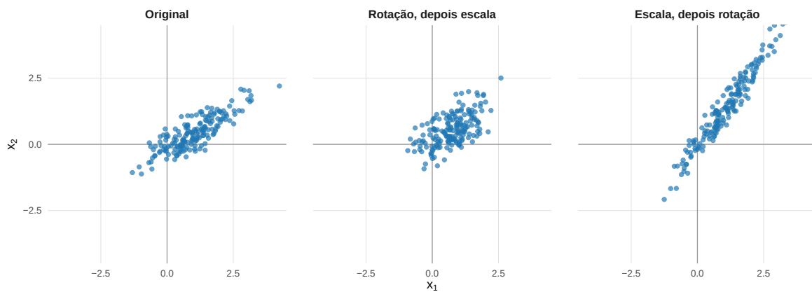
Figura 4.3: Efeito da ordem na composição de uma rotação e de um escalonamento não uniforme.
