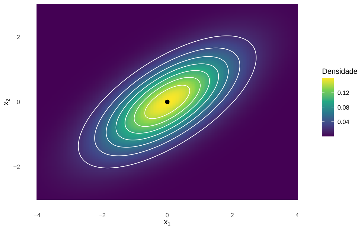
Figura 10.1: Mapa de densidade e curvas de nível de uma distribuição normal bivariada.
