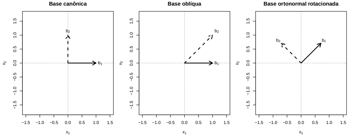
Figura 4.3: Comparação entre a base canônica, uma base oblqua e uma base ortonormal rotacionada de \mathbb{R}^2 .
