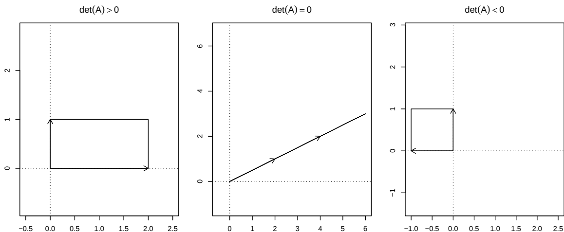
Figura 3.1: Interpretação geométrica do determinante em duas dimensões.
