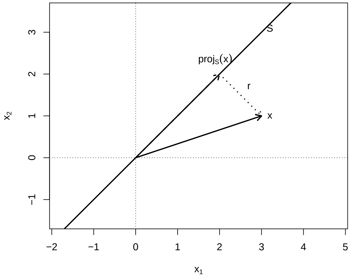
Figura 4.5: Decomposição de um vetor em sua projeção sobre um subespaço e em um resíduo ortogonal.
