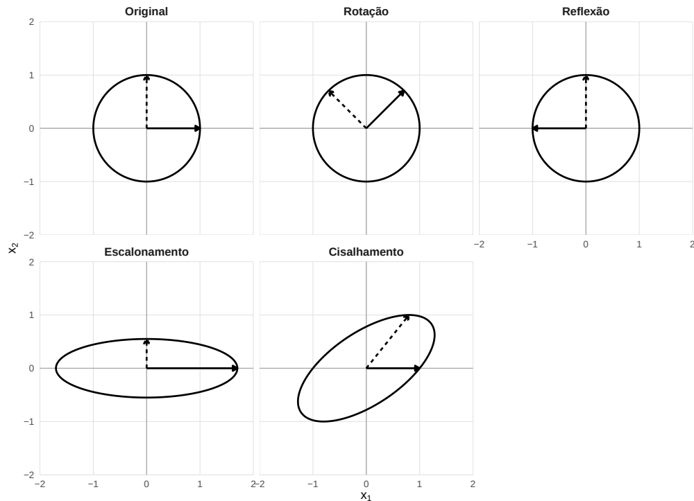
Figura 5.6: Efeito de transformações ortogonais e não ortogonais sobre a circunferência unitária e duas direções ortogonais.
