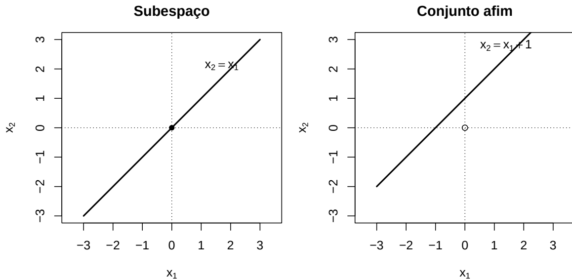
Figura 4.1: Comparação entre um subespaço de \mathbb{R}^2 e uma reta afim.
