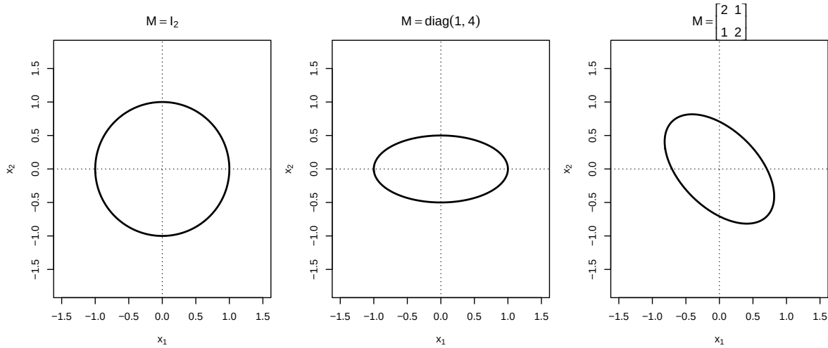
Figura 4.4: Curvas de norma unitária para diferentes produtos internos em \mathbb{R}^2 .
