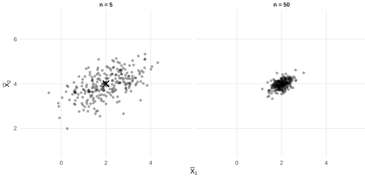
Figura 11.1: Vetores de médias amostrais em amostras bivariadas de tamanhos 5 e 50.
