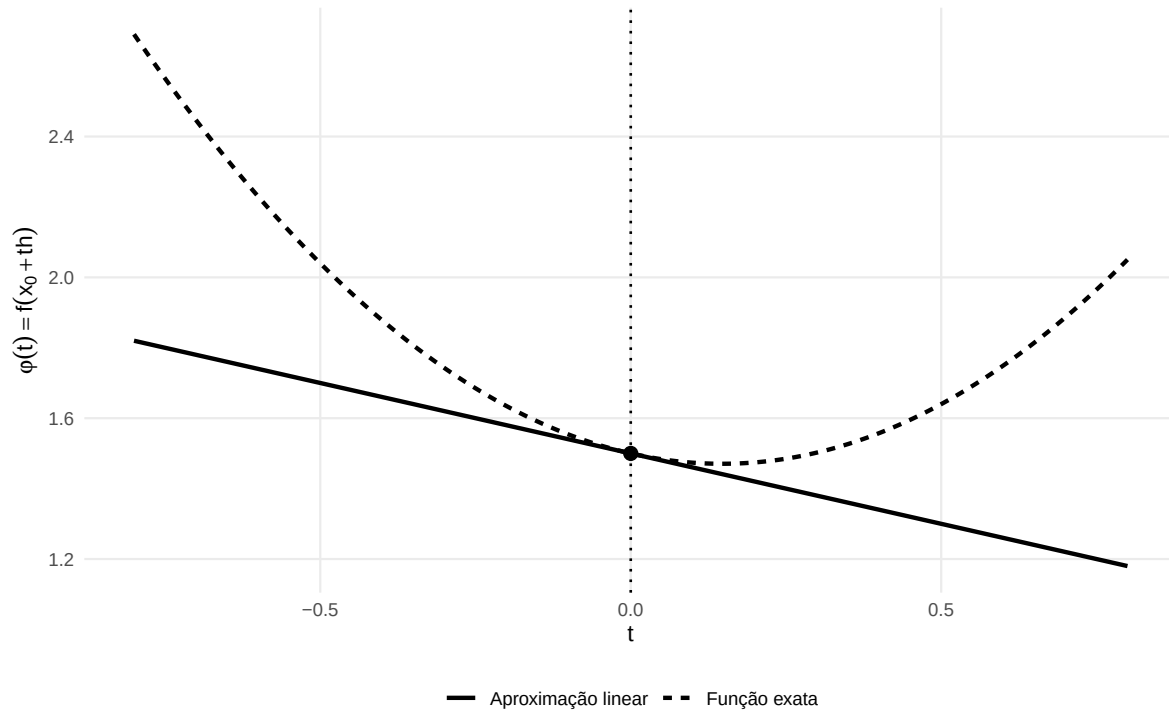
Figura 8.1: Função exata ao longo de uma direção e aproximação linear no ponto t = 0 .
