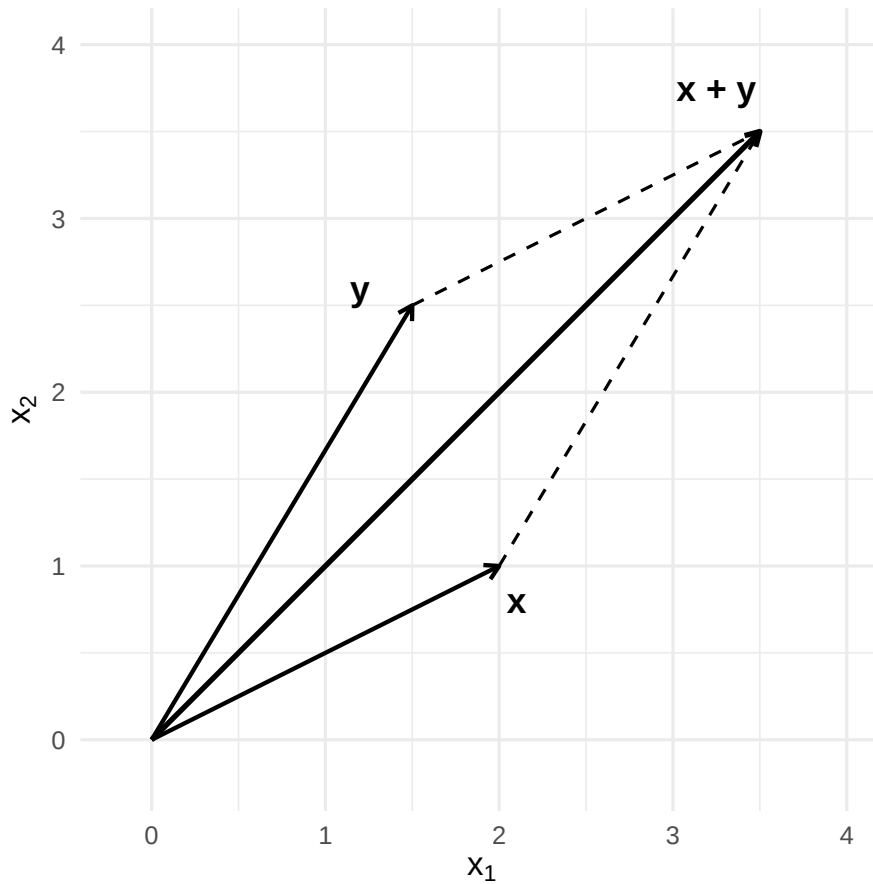
Figura 2.3: Soma de vetores pela regra do paralelogramo.
