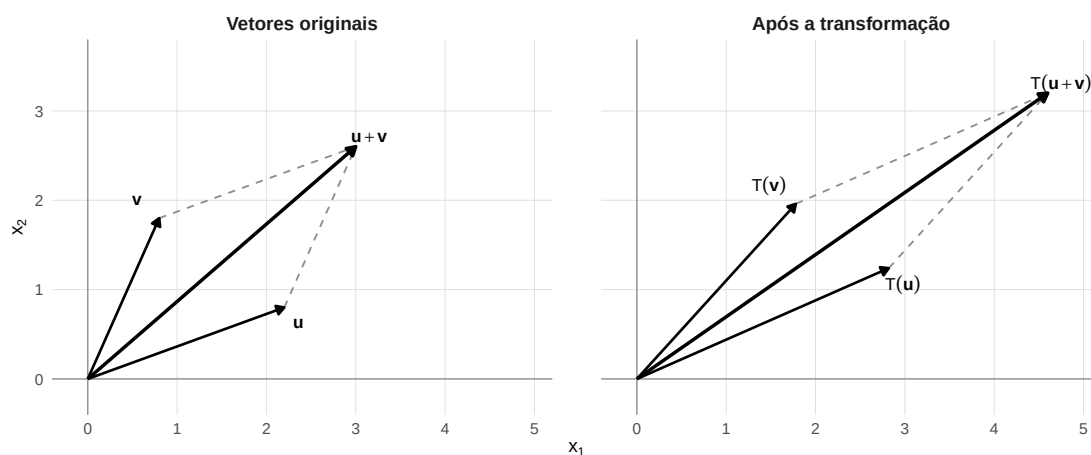
Figura 5.1: Preservação da soma de vetores por uma transformação linear.
