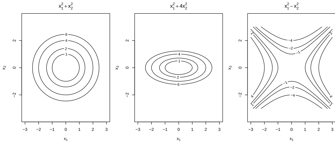
Figura 3.2: Curvas de nível de formas quadráticas em duas dimensões.
