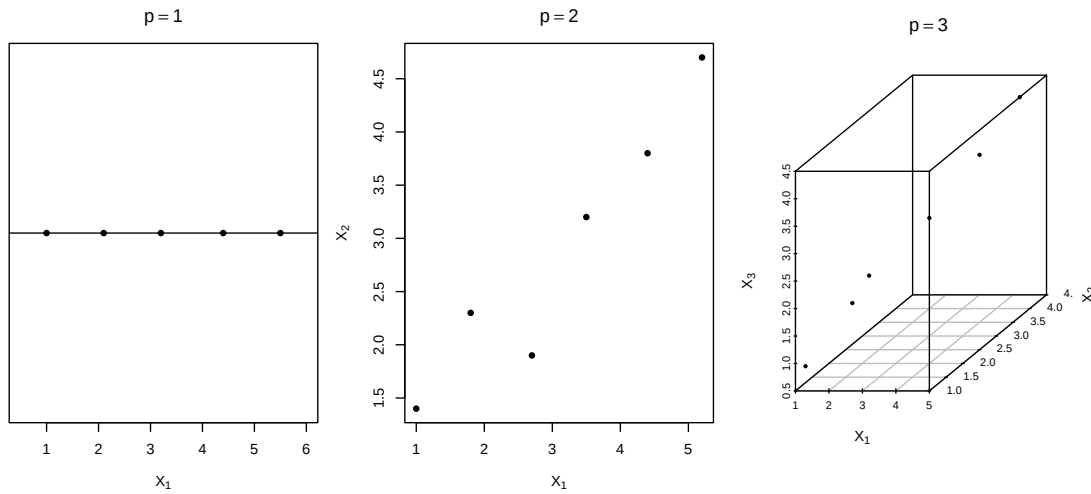
Figura 2.1: Representação de observações em espaços de uma, duas e três dimensões.
