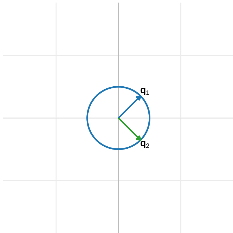
Circunferência unitária
