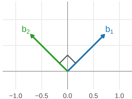
Base ortonormal rotacionada
