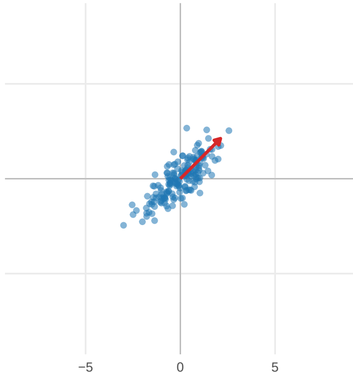
Correlações
