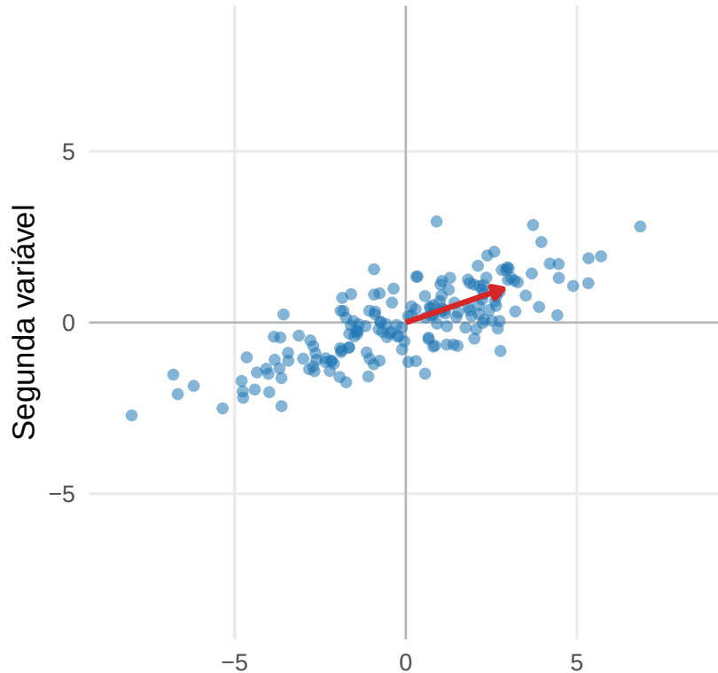
Covariâncias
