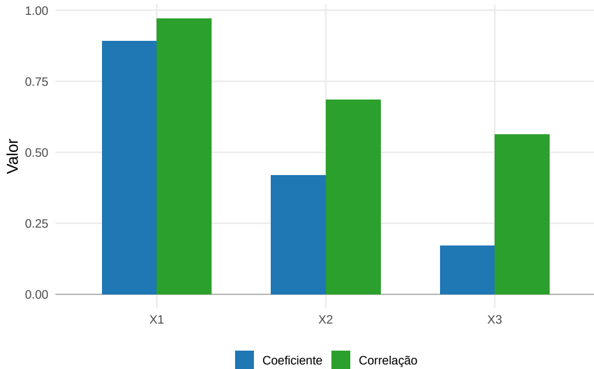
Figura 14.5: Os coeficientes definem a direção da componente, enquanto as correlações medem a associação de cada variável com a componente.
