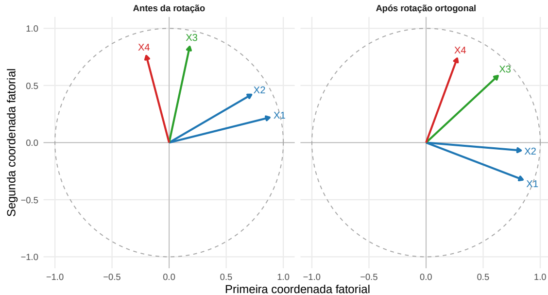
Figura 15.4: Uma rotação ortogonal modifica as coordenadas das cargas, mas preserva comprimentos, produtos internos, communalidades e a matriz de covariâncias comuns.
