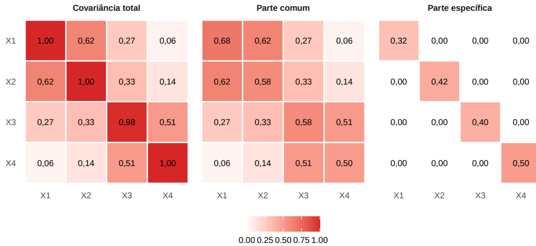
Figura 15.3: Decomposição de uma matriz de covariâncias em estrutura comum, produzida pelas cargas fatoriais, e estrutura específica diagonal.
