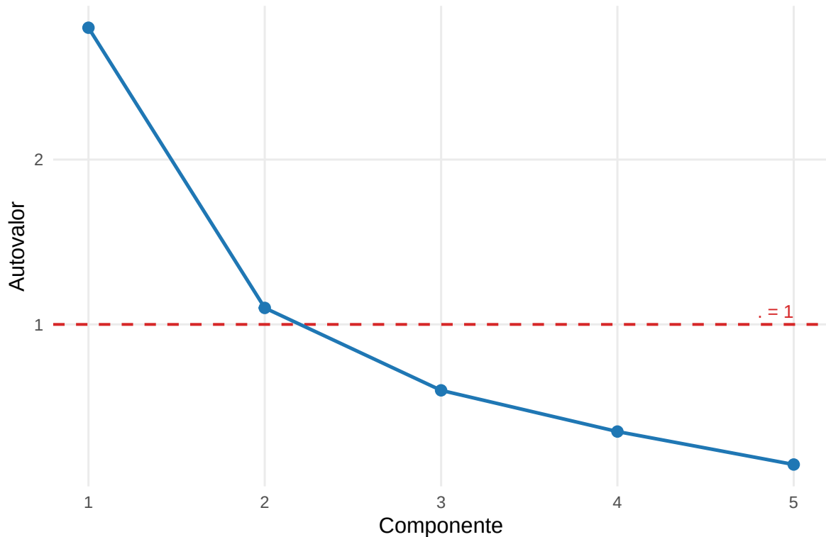
Figura 14.5: Gráfico de declive dos autovalores. A linha tracejada indica a referência autovalor igual a 1 para uma ACP baseada em correlações.
