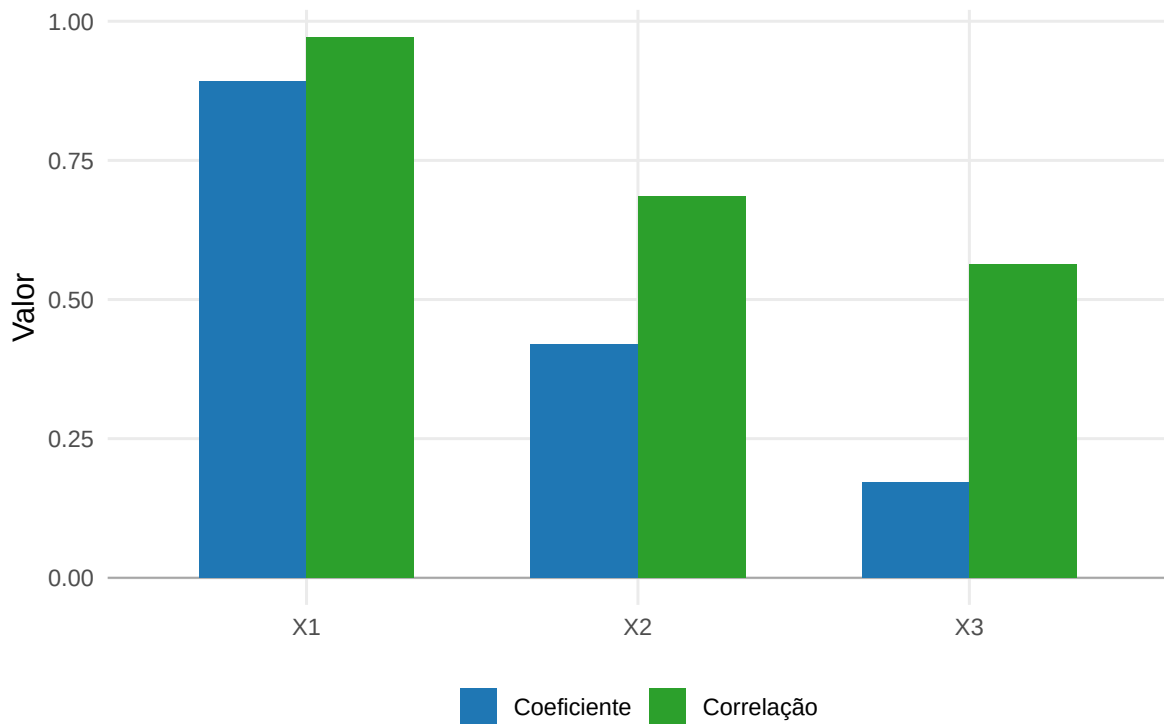
Figura 14.6: Os coeficientes definem a direção principal associada à componente, enquanto as correlações medem a associação linear de cada variável com essa componente.
