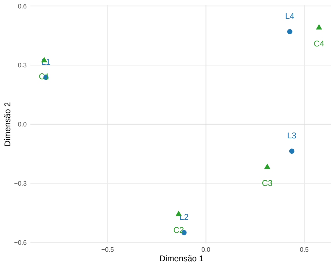
Figura 17.3: Representação conjunta das categorias de linhas e colunas nas duas primeiras dimensões. As distâncias dentro de cada nuvem são representadas no subespaço exibido; a distância entre uma linha e uma coluna não corresponde, em geral, a uma distância qui-quadrado.
