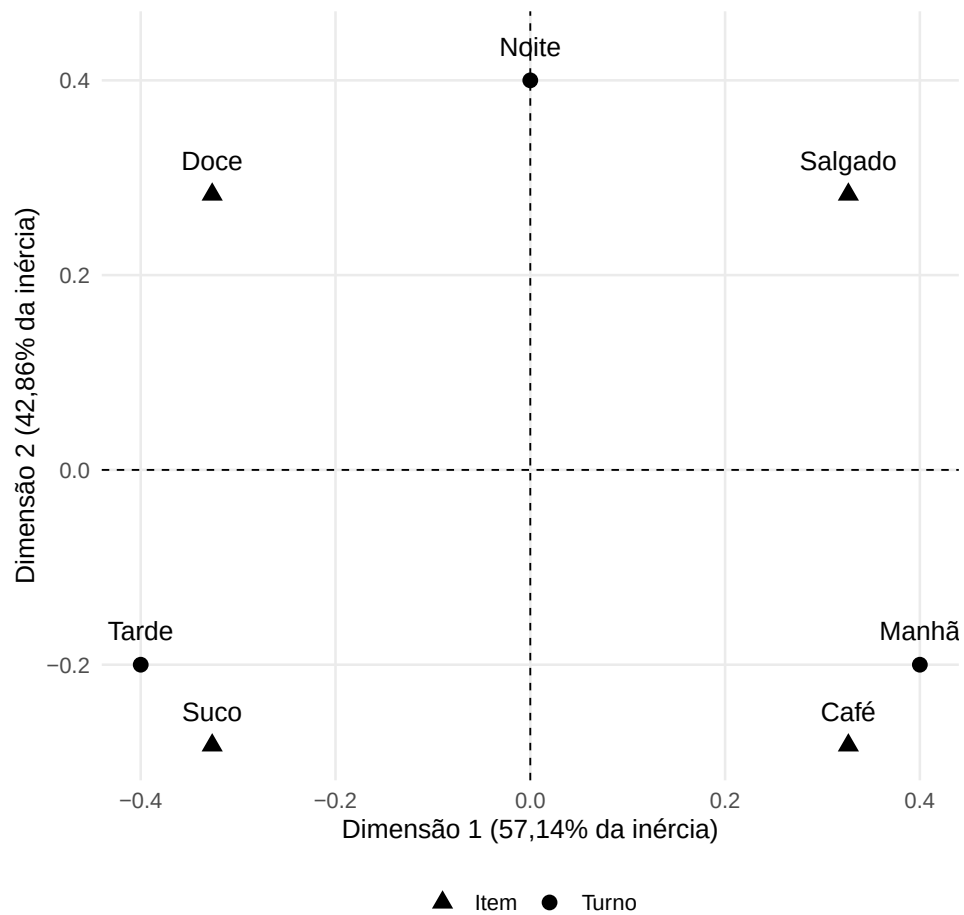
Figura 17.1: Representação das categorias de linha e de coluna nas duas dimensões da Análise de Correspondência.
