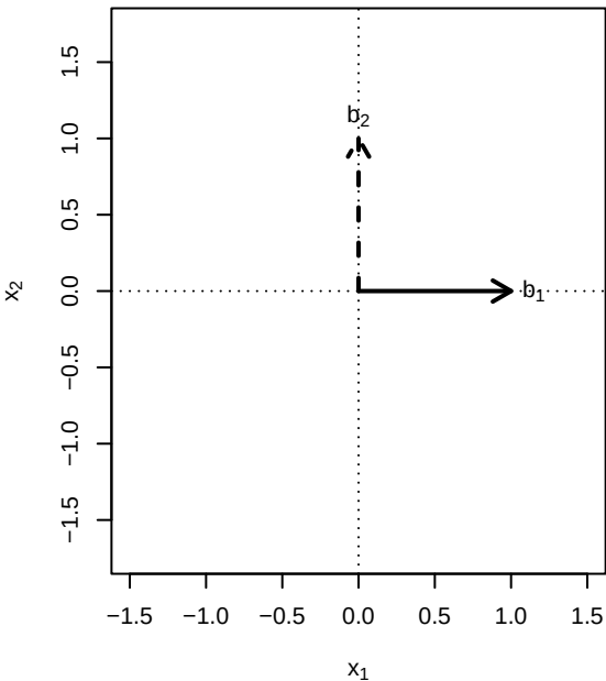
Base canônica
