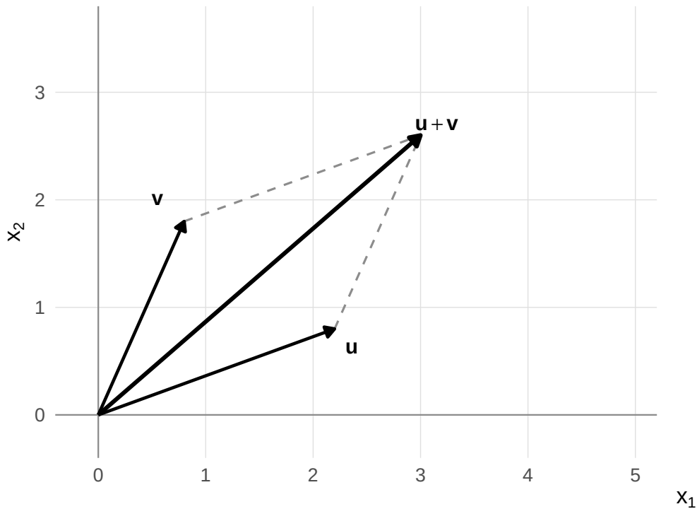
Vetores originais
