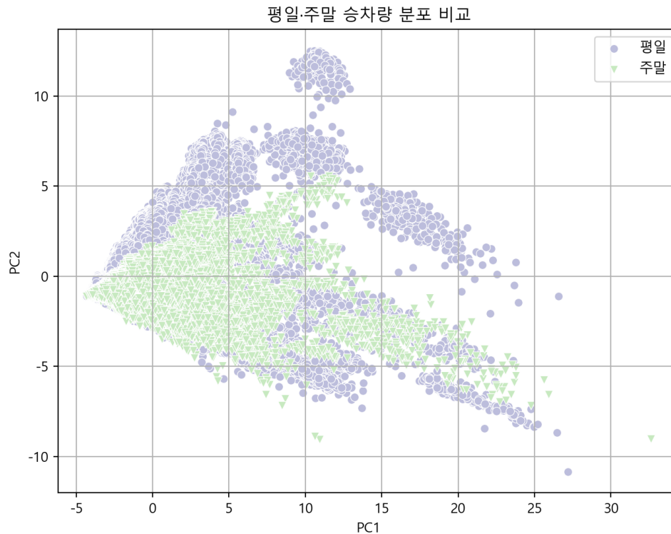
[그림 A-5-7] 평일·주말 승차량 분포 비교
