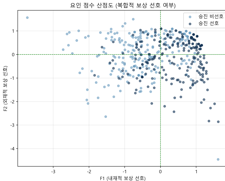
[그림 A-5-10] 요인 점수 산점도
