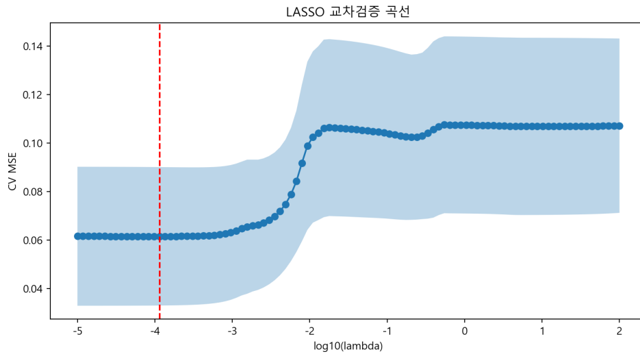
[그림 A-5-4] 라쏘 교차검증 곡선
