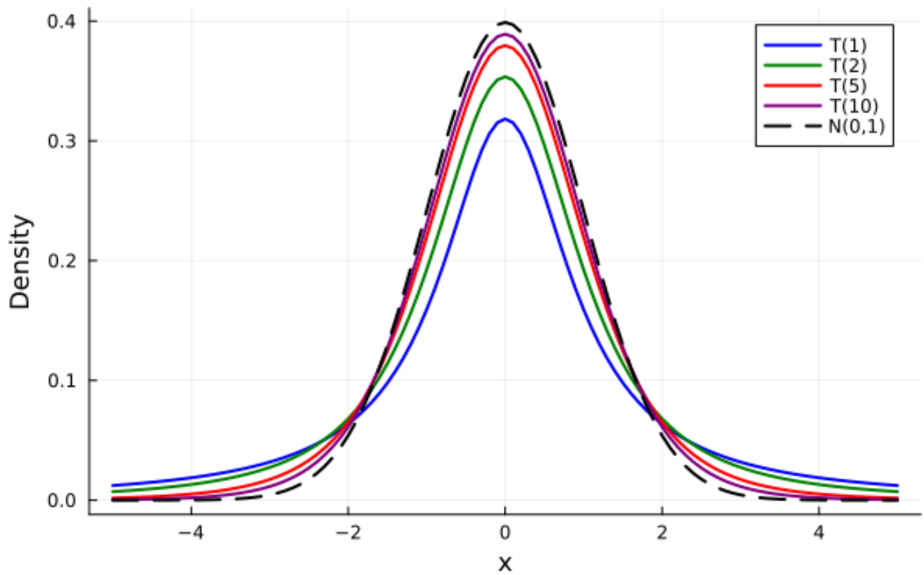
FIGURE 26.1 – Densité de plusieurs lois de Student.
