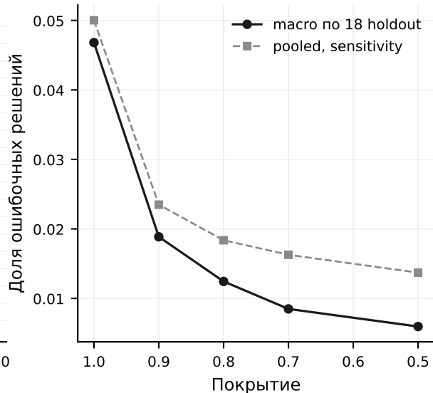
Risk-coverage: порог не выбран
