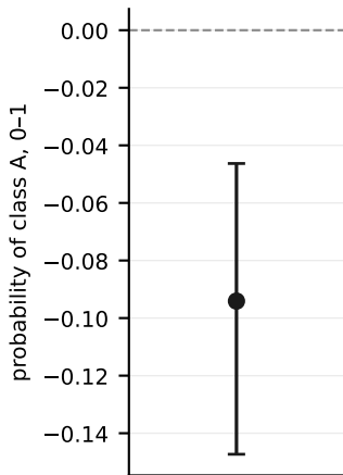
2. classifier P2b
