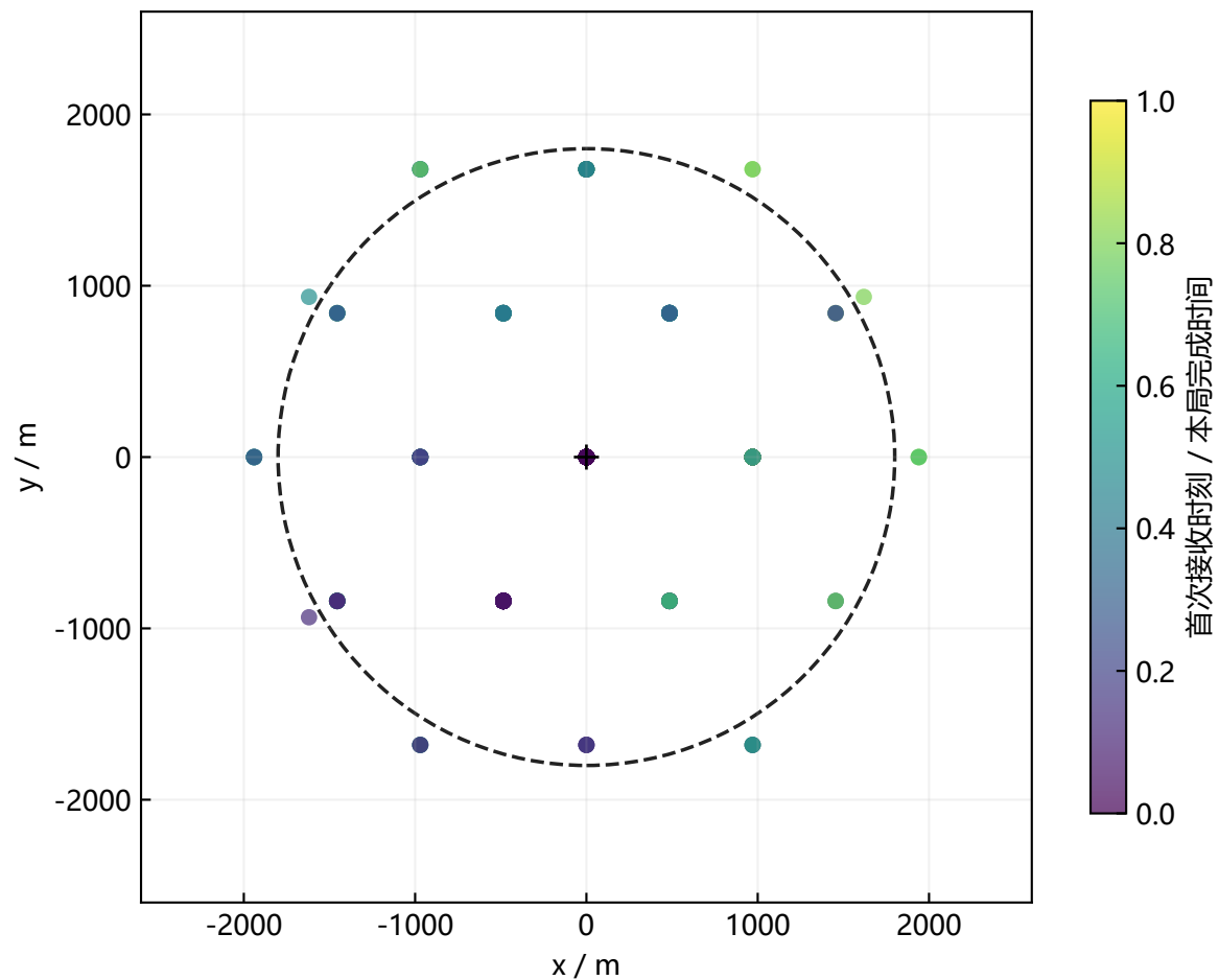
Q4 官方首次成功接收测点 · 358个源
