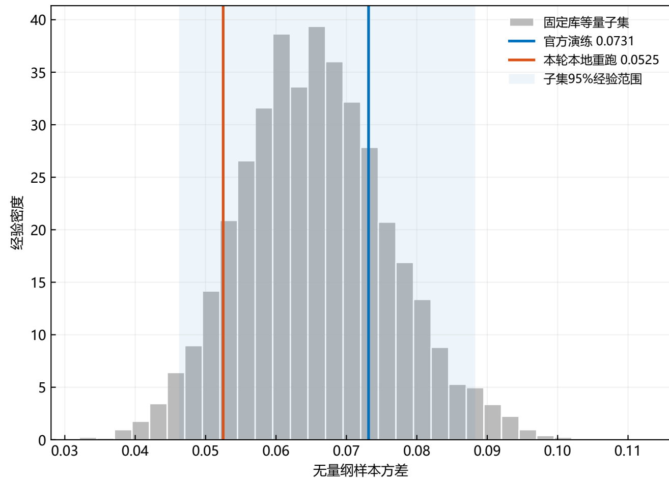
Q4：按官方源数构成抽取5000次
