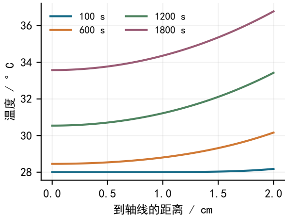
(a) 温度的径向分布
