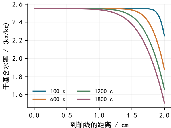
(b) 含水率的径向分布
