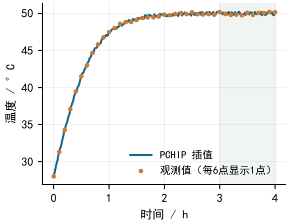
(a) 烘房温度
