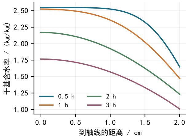
(b) 含水率的径向分布
