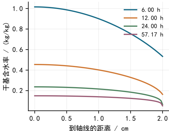
(b) 代表时刻的物理坐标剖面
