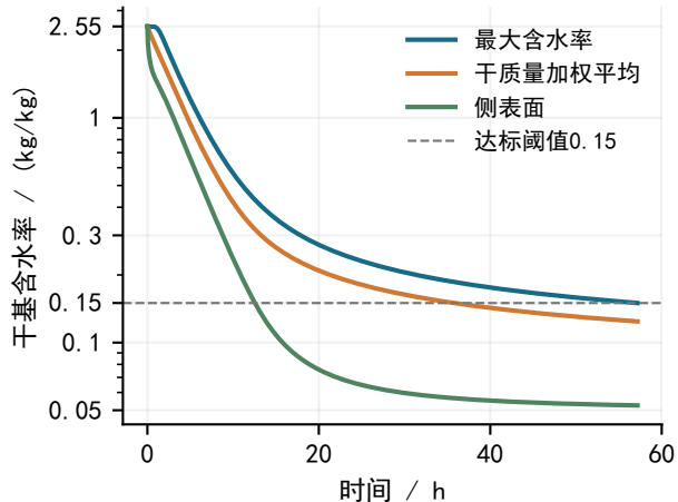
(a) 干燥过程（纵轴为对数）
