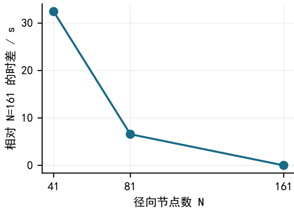
(a) 空间加密 (时间步长1s)
