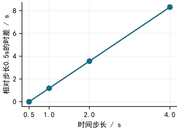
(b) 时间加密 (81节点)
