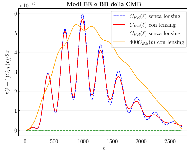
Figure 4: Confronto tra i vari modi di polarizzazione della CMB, con e senza le correzioni di lensing.
