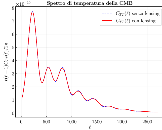
Figure 2: Confronto tra C_{TT} con e senza le correzioni di lensing.
