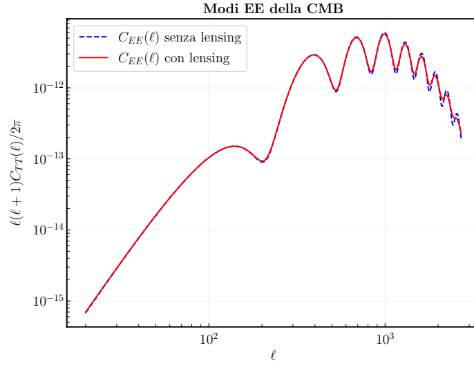
Figure 3: Confronto tra C_{EE} con e senza le correzioni di lensing.
