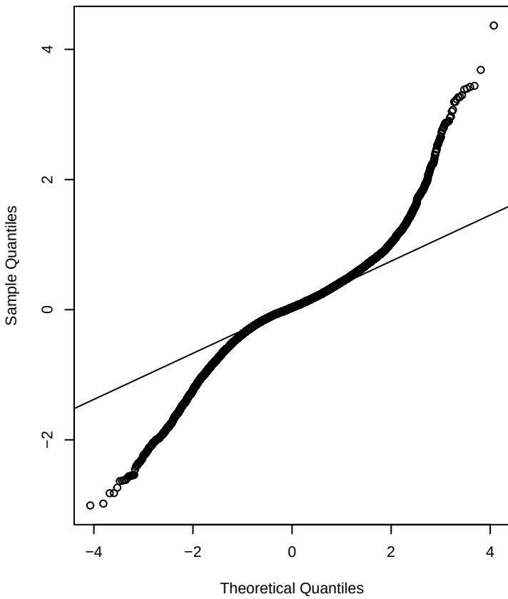
K_corr - Q-Q Plot
