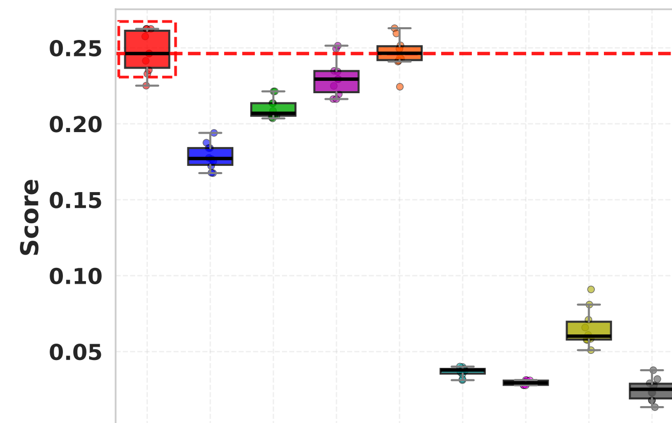
Cell-type ASW
