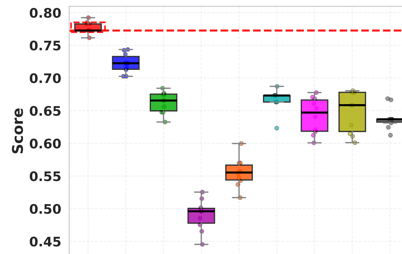
NMI
