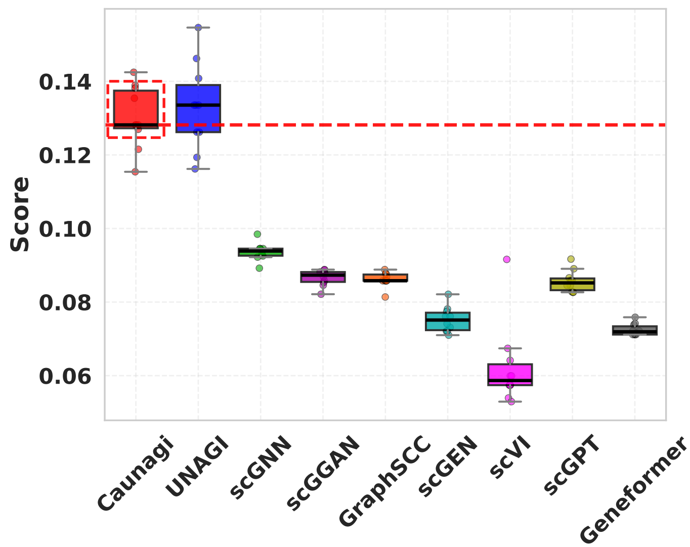
Isolated F1
