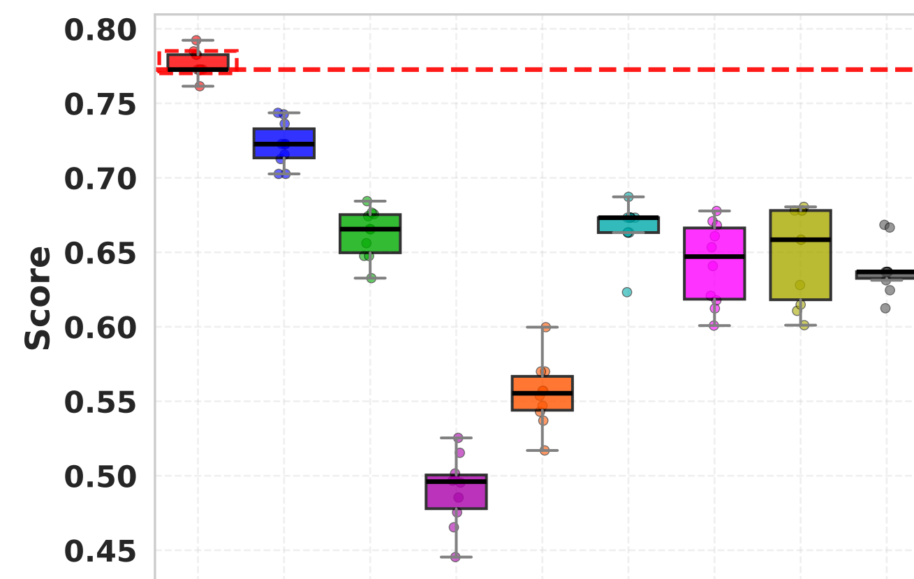
NMI
