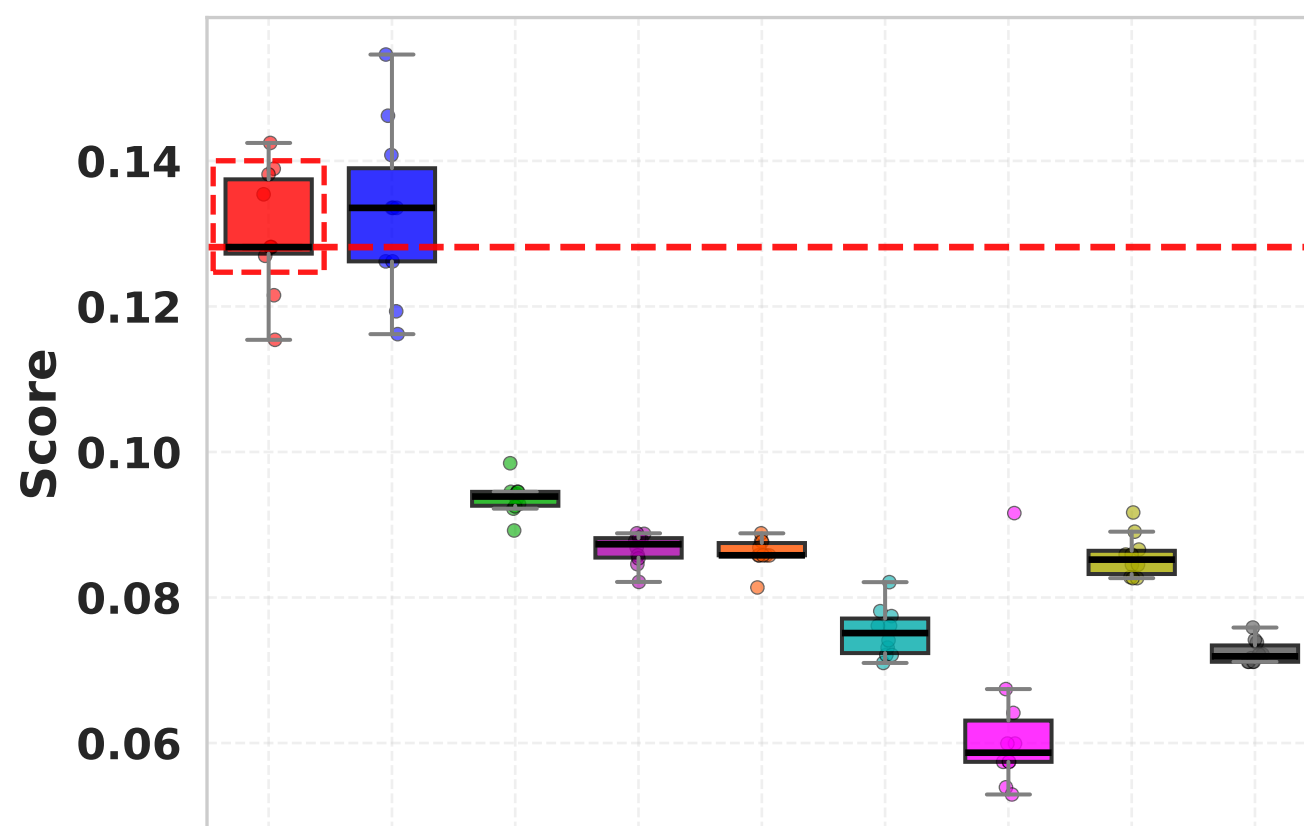
Isolated F1
