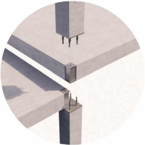
betonnen casco
