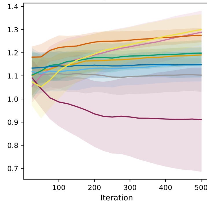
(g) BRAF
