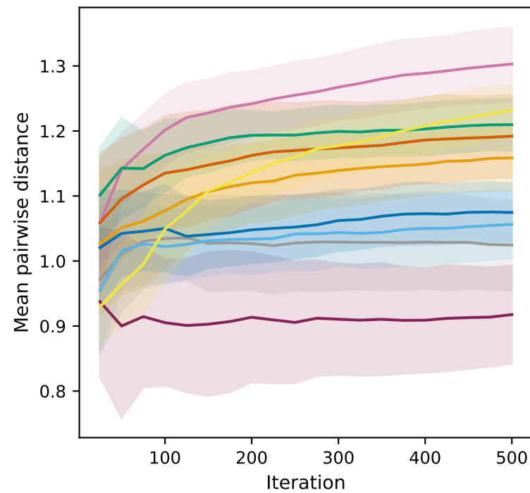
(e) DHFR
