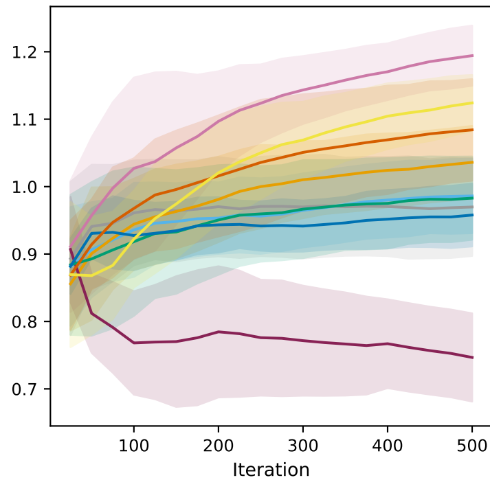
(f) JAK3
