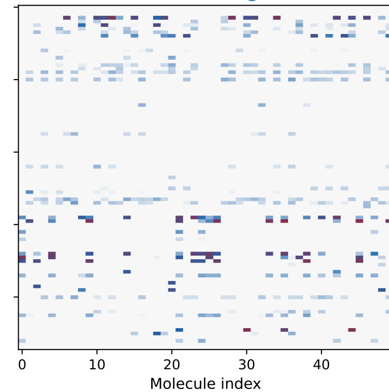
Genetic Alg.
