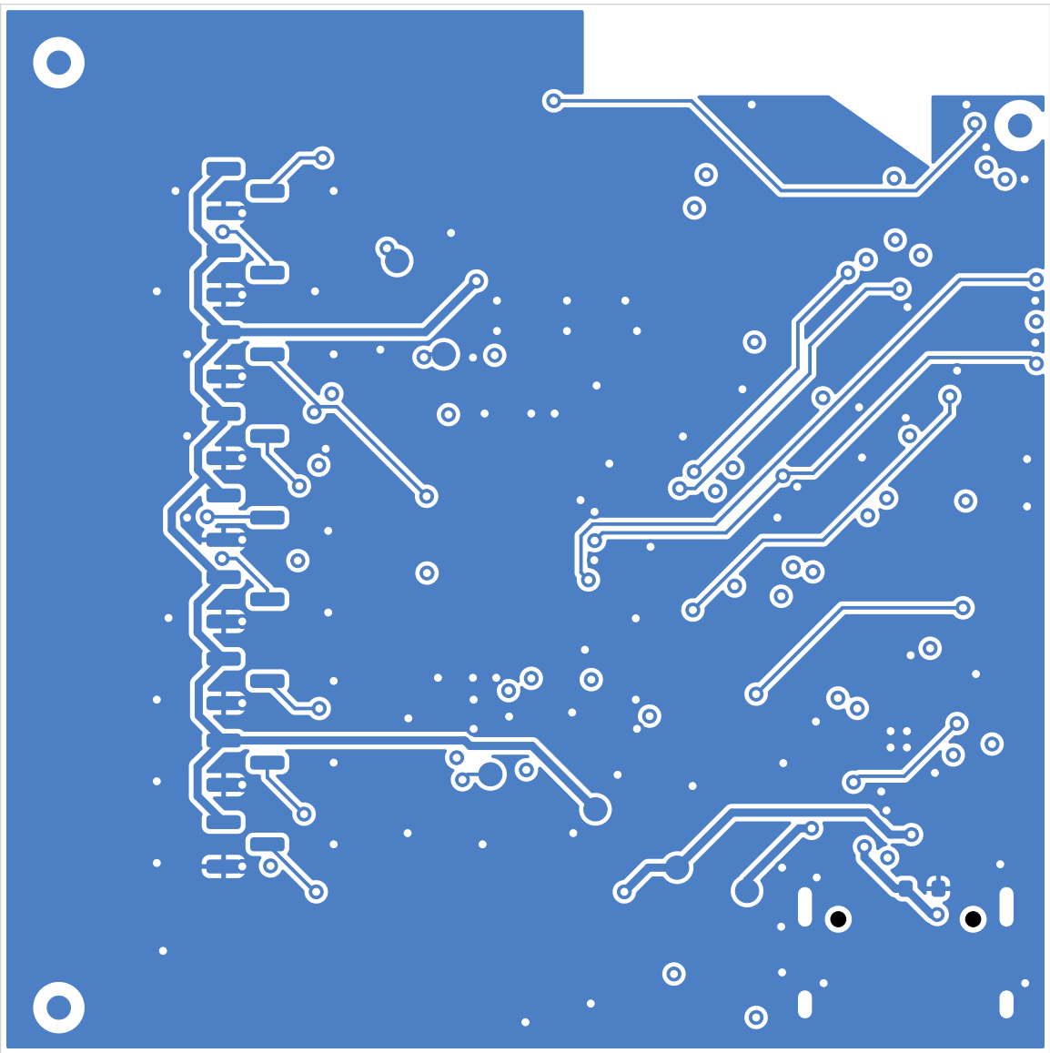
B.Cu
