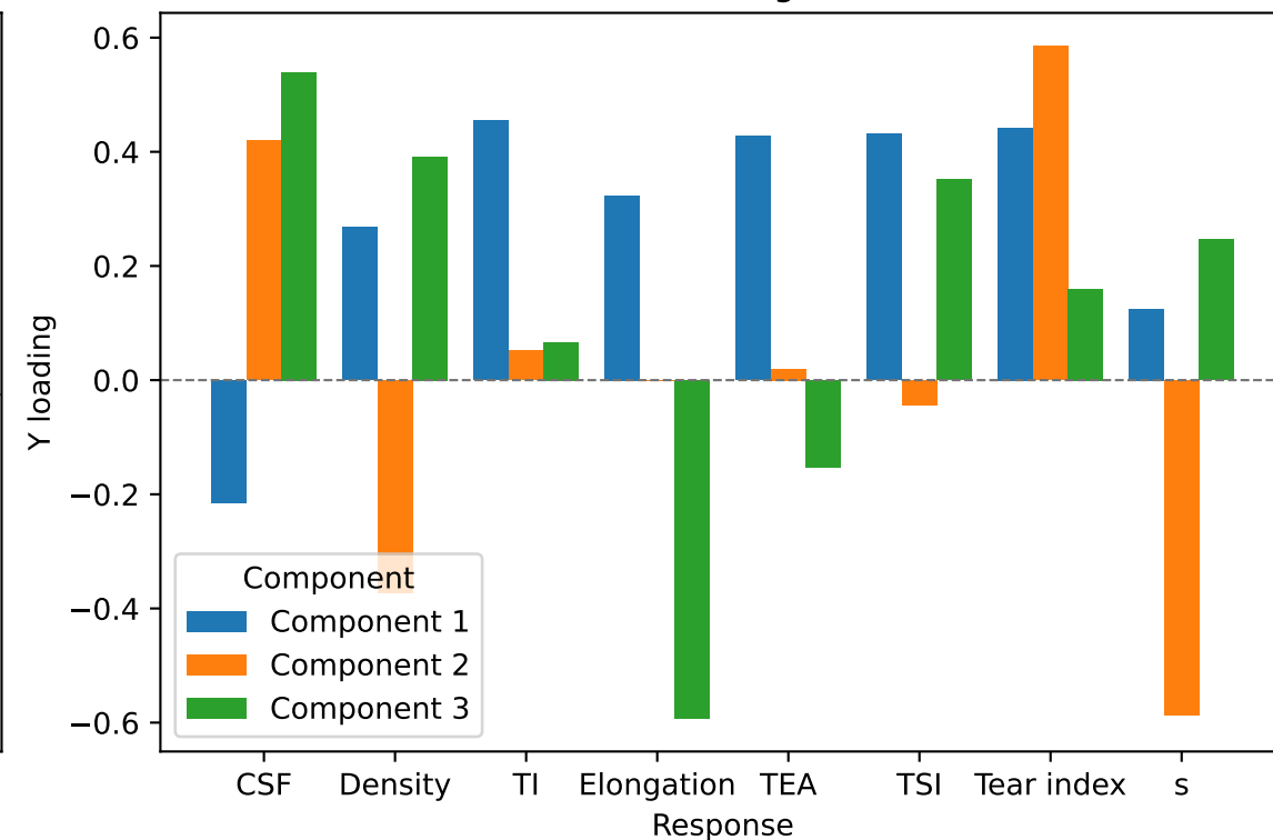
Y loadings
