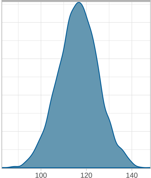
b_IsWordFALSE
