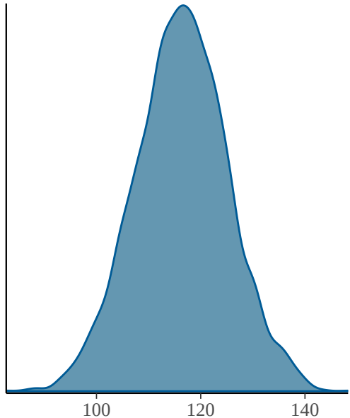
b_IsWordFALSE
