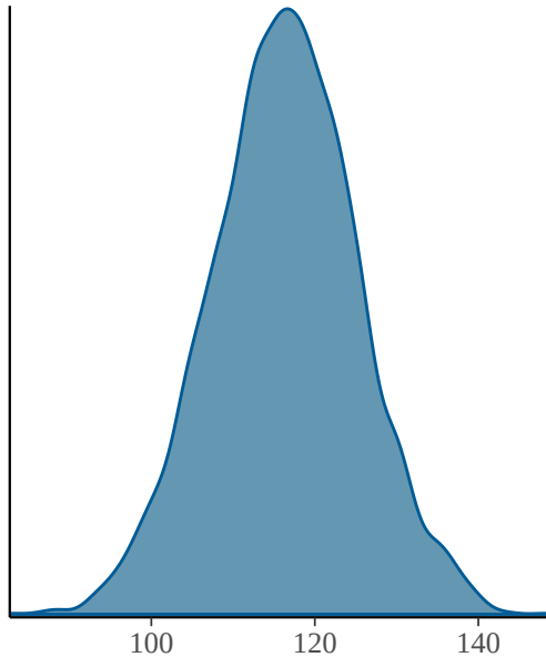
b_IsWordFALSE
