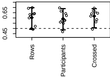
ROC AUC
