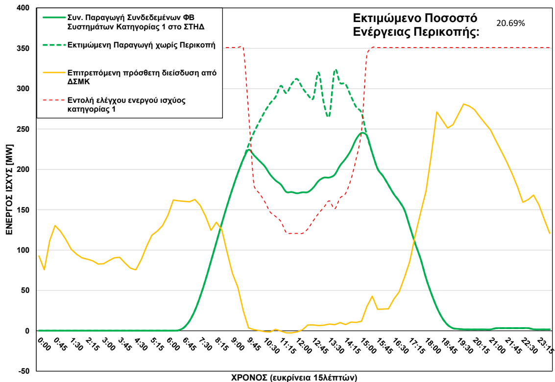
ΦΒ Παραγωγή στο ΣΤΗΔ στις 31/08/2026 (ώρα περικοπής: 09:45 - 15:00)
