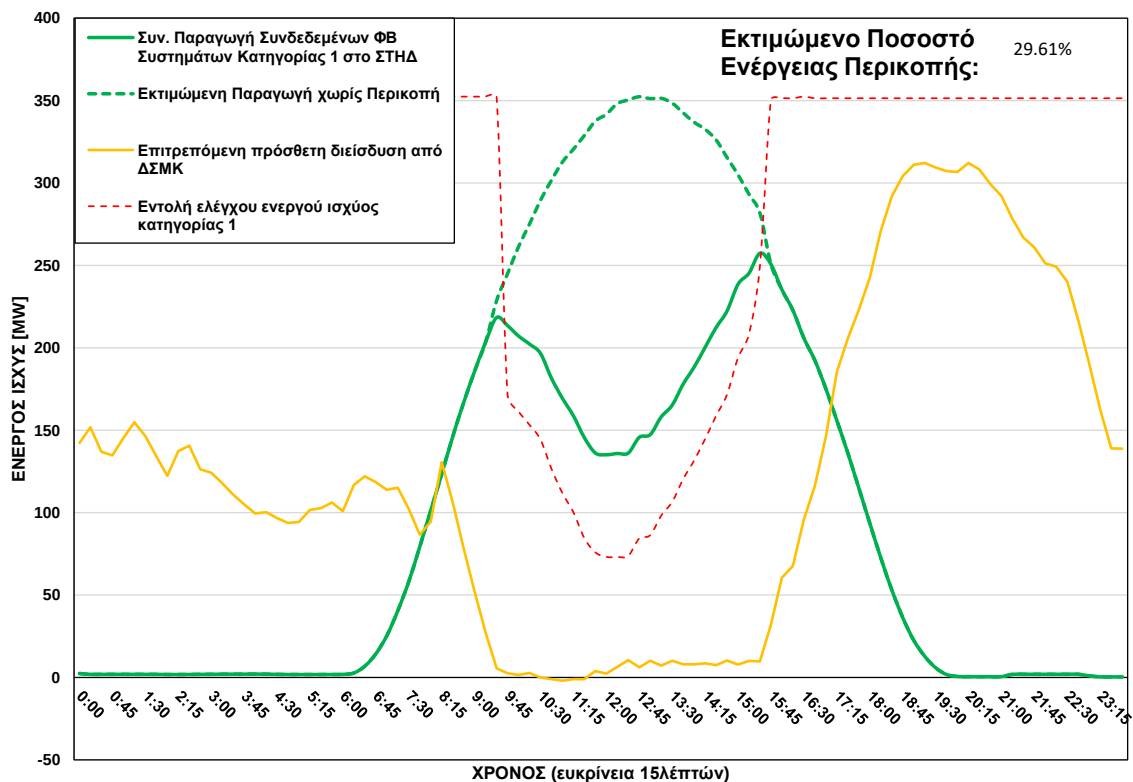
ΦΒ Παραγωγή στο ΣΤΗΔ στις 04/08/2026 (ώρα περικοπής: 09:30 - 15:30)
