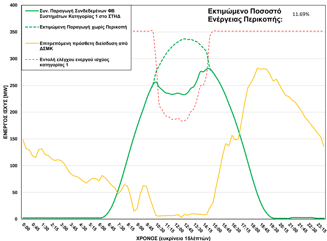
ΦΒ Παραγωγή στο ΣΤΗΔ στις 10/08/2026 (ώρα περικοπής: 10:30 - 14:30)
