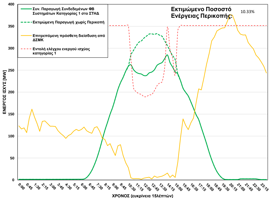
ΦΒ Παραγωγή στο ΣΤΗΔ στις 11/08/2026 (ώρα περικοπής: 10:45 - 15:00)
