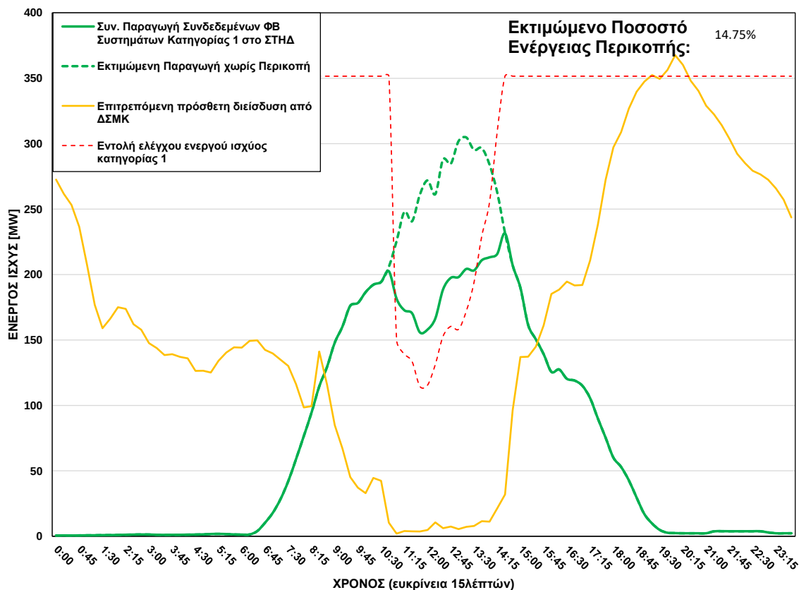
ΦΒ Παραγωγή στο ΣΤΗΔ στις 14/08/2026 (ώρα περικοπής: 10:45 - 14:15)
