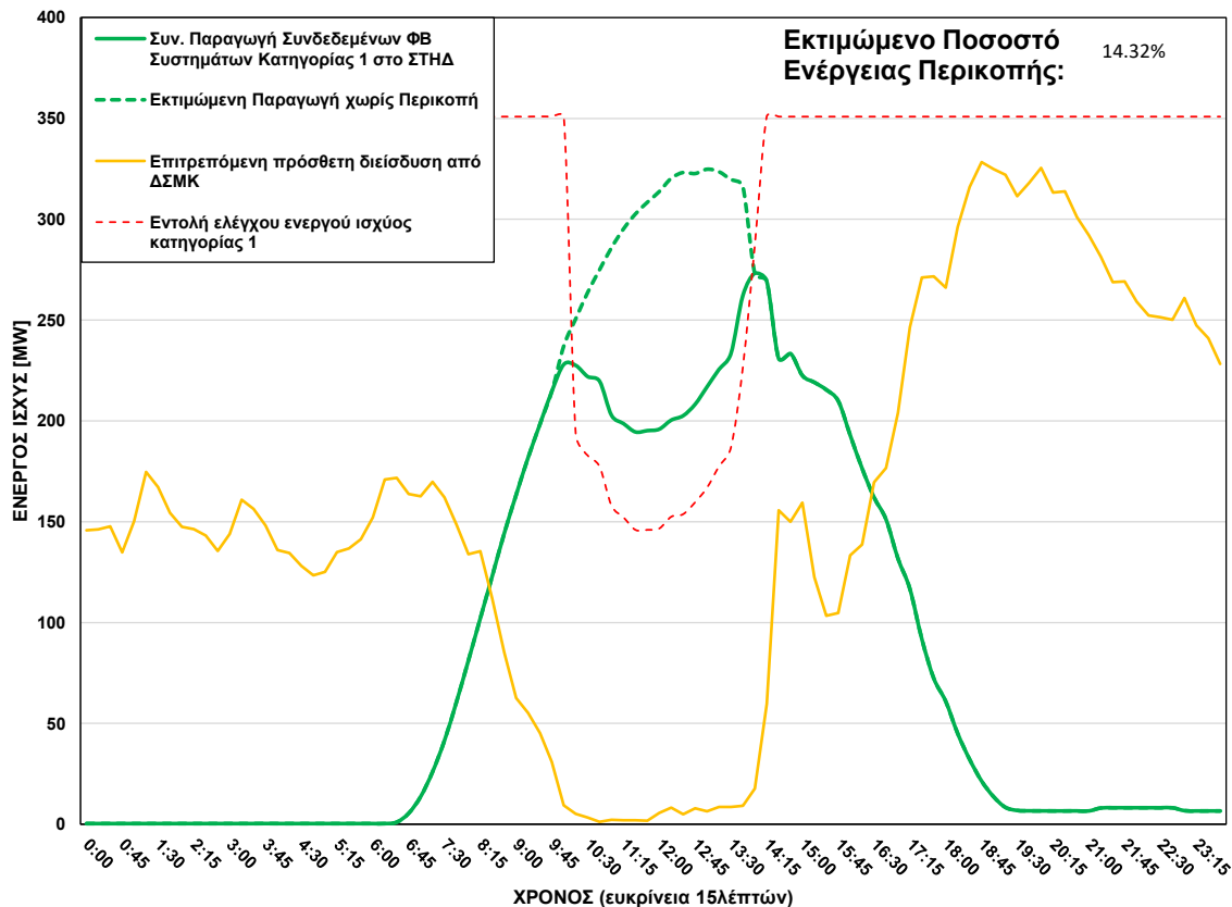
ΦΒ Παραγωγή στο ΣΤΗΔ στις 28/08/2026 (ώρα περικοπής: 10:00 - 13:45)
