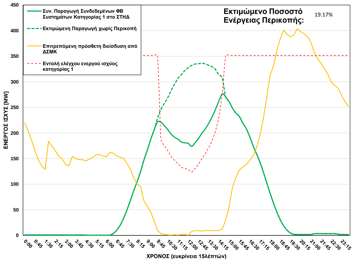
ΦΒ Παραγωγή στο ΣΤΗΔ στις 12/08/2026 (ώρα περικοπής: 09:45 - 14:30)
