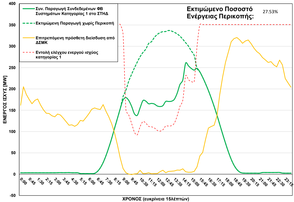
ΦΒ Παραγωγή στο ΣΤΗΔ στις 26/08/2026 (ώρα περικοπής: 09:00 - 15:15)
