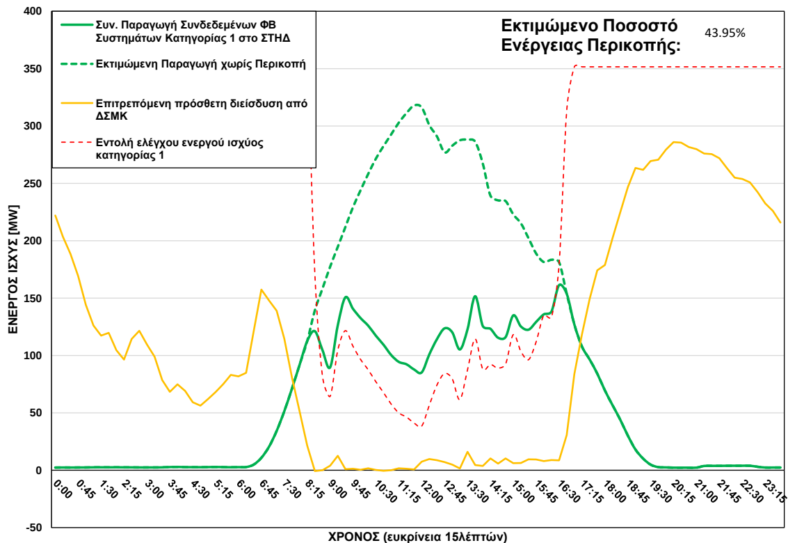
ΦΒ Παραγωγή στο ΣΤΗΔ στις 15/08/2026 (ώρα περικοπής: 08:30 - 16:30)
