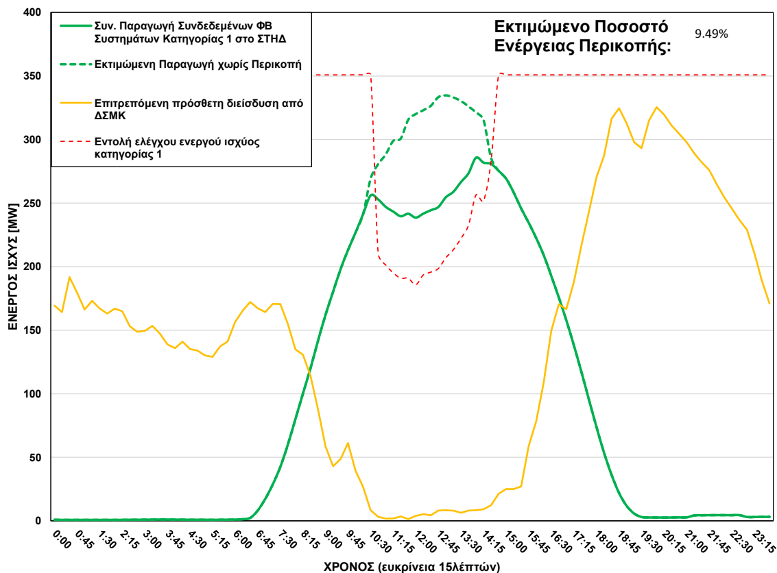
ΦΒ Παραγωγή στο ΣΤΗΔ στις 25/08/2026 (ώρα περικοπής: 10:30 - 14:15)
