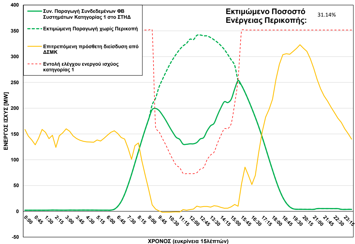
ΦΒ Παραγωγή στο ΣΤΗΔ στις 20/08/2026 (ώρα περικοπής: 09:15 - 15:15)
