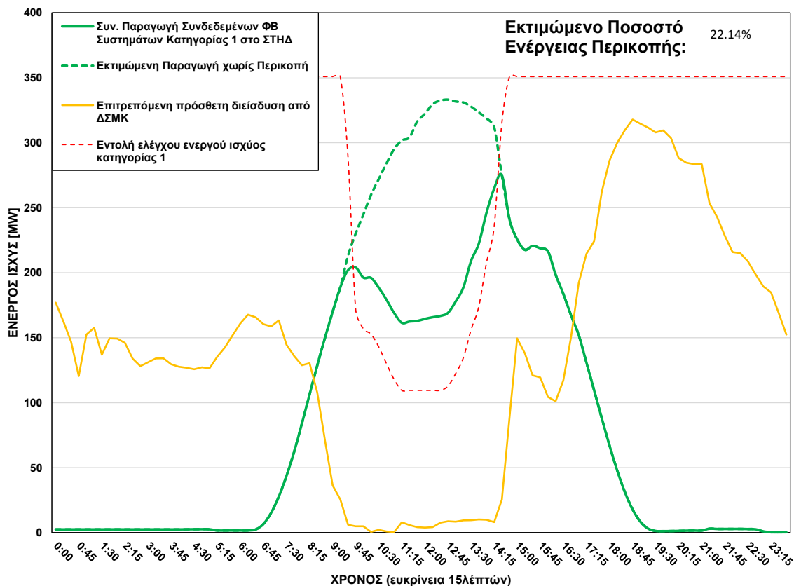
ΦΒ Παραγωγή στο ΣΤΗΔ στις 27/08/2026 (ώρα περικοπής: 09:30 - 14:15)
