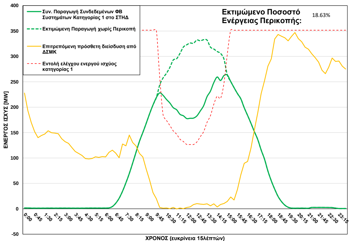
ΦΒ Παραγωγή στο ΣΤΗΔ στις 13/08/2026 (ώρα περικοπής: 10:00 - 14:45)
