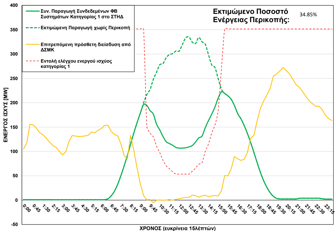
ΦΒ Παραγωγή στο ΣΤΗΔ στις 19/08/2026 (ώρα περικοπής: 09:15 - 15:15)
