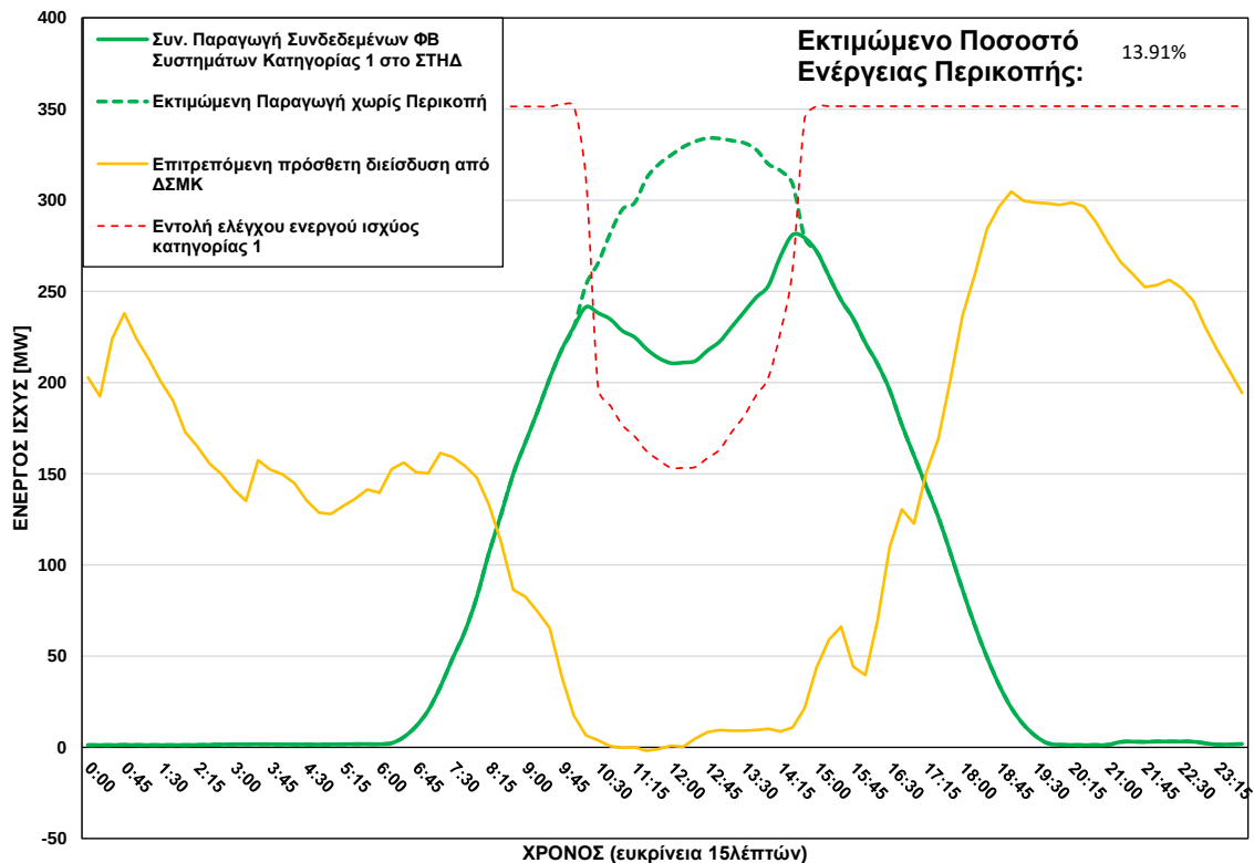
ΦΒ Παραγωγή στο ΣΤΗΔ στις 07/08/2026 (ώρα περικοπής: 10:15 - 14:30)
