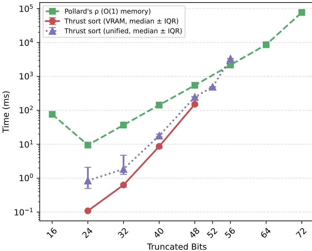
MD5
