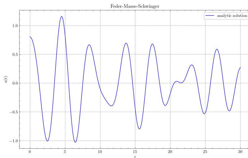
Figure 58: Analytische Lösung des Feder-Masse-Schwingers
