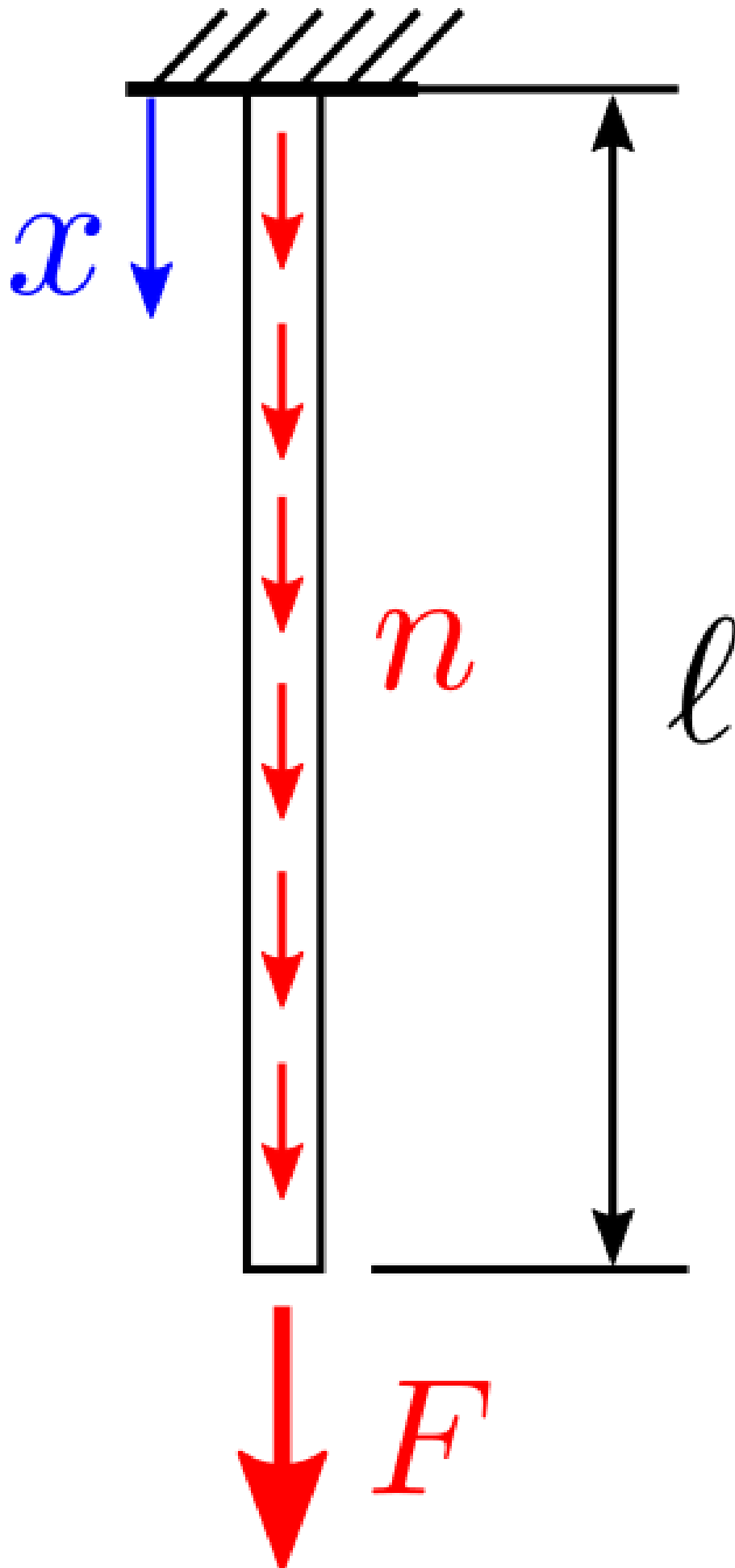
Figure 18: Stab unter Eigengewicht und externer Kraft.
