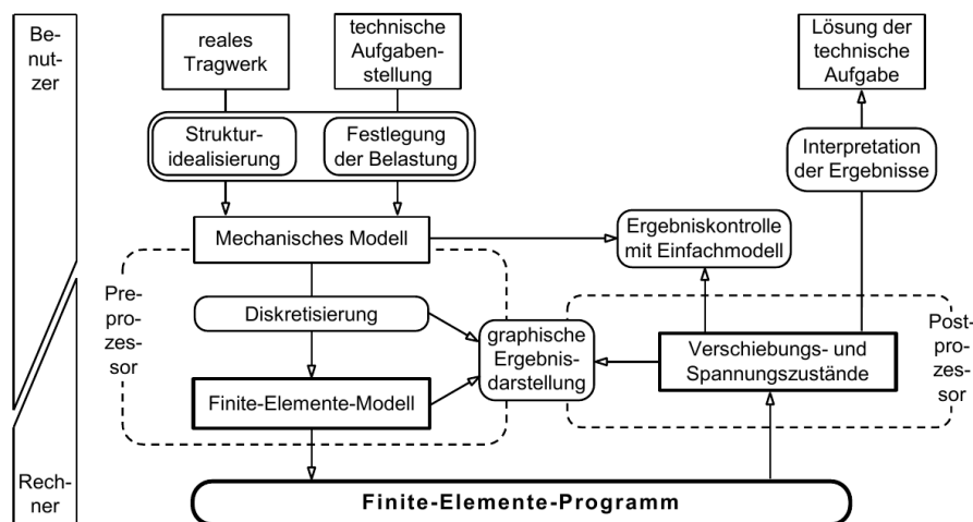
Figure 1: Einordnung numerischer Simulation in den Konstruktionsprozess nach Knothe and Wessels [1991]
