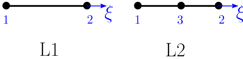
Figure 42: 1D-Elemente mit linearer und quadratischer Ansatzfunktion
