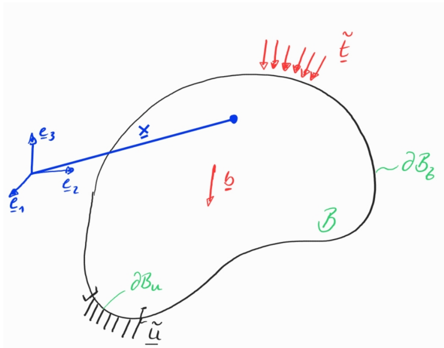
Figure 8: Körper \mathcal{B} unter Einwirkung der externen Oberflächenkraft \tilde{t} und der Volumenlast b
