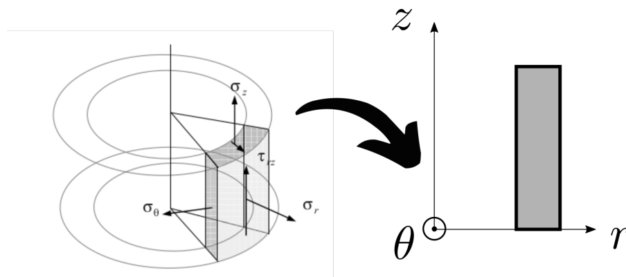
Figure 13: Rotationssymmetrischer Körper im Zylinderkoordinatensystem \{r, z, \theta\} . Nach Chaves [2013]
