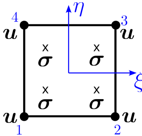
Figure 55: Unterschied zwischen primären und sekundären Größen im Postprocessing.
