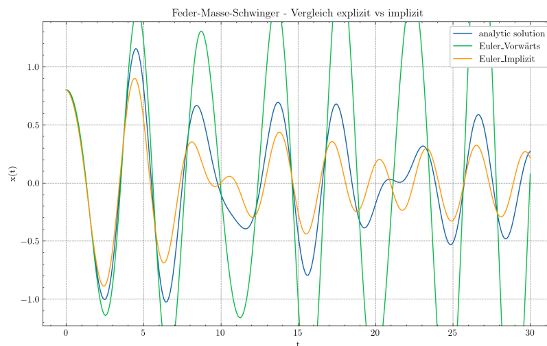
Figure 60: Analytische und numerische Losung des Feder-Masse-Schwingers im Vergleich.
