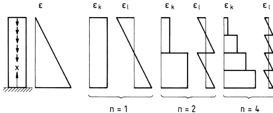
Figure 39: Mit steigender Elementanzahl wird der konstante Term der Schnittkraft dominant (Knothe and Wessels [1991]).
