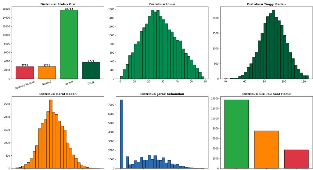
Gambar 3. Eksplorasi distribusi data (EDA).
