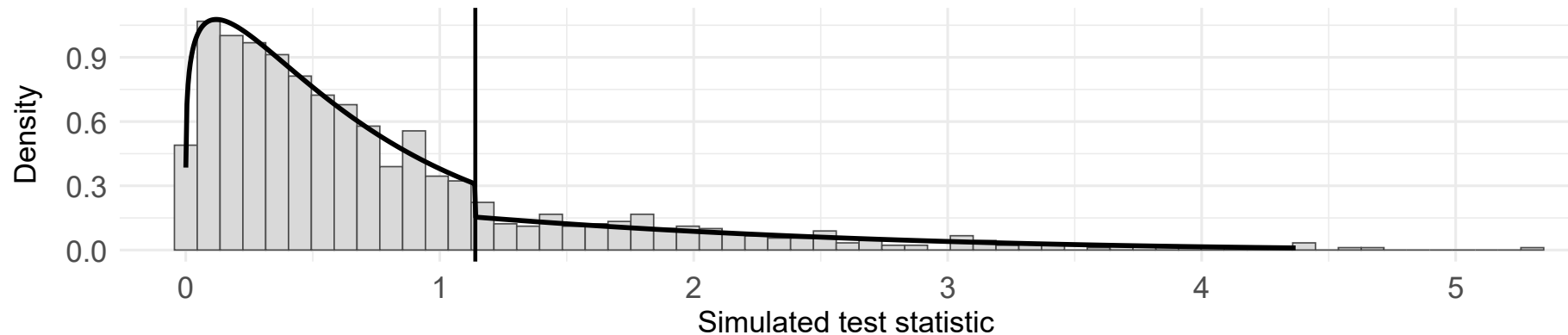
(d) Gamma-GPD ( k_0 = 250 )
