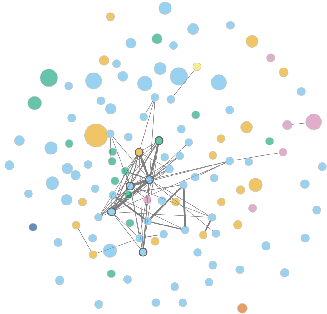
EBF
