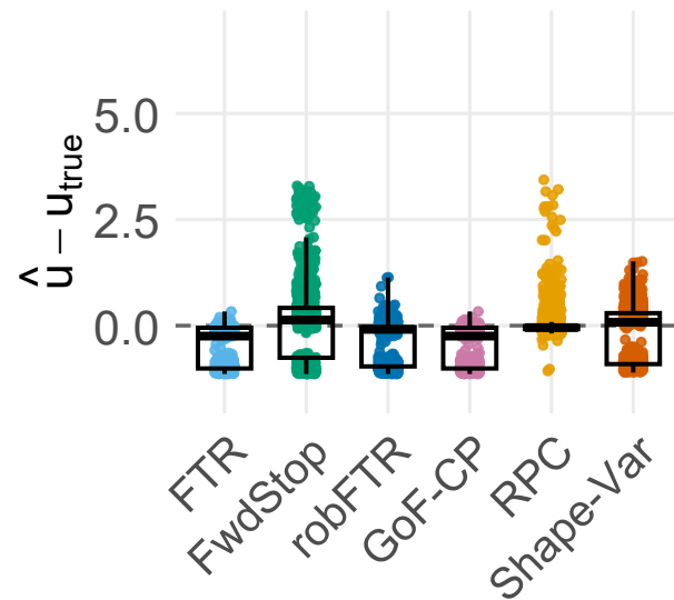
Gamma-GPD
