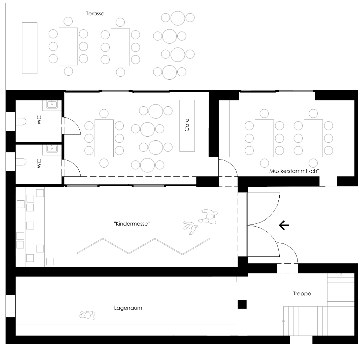
Erdgeschoss M1:100
