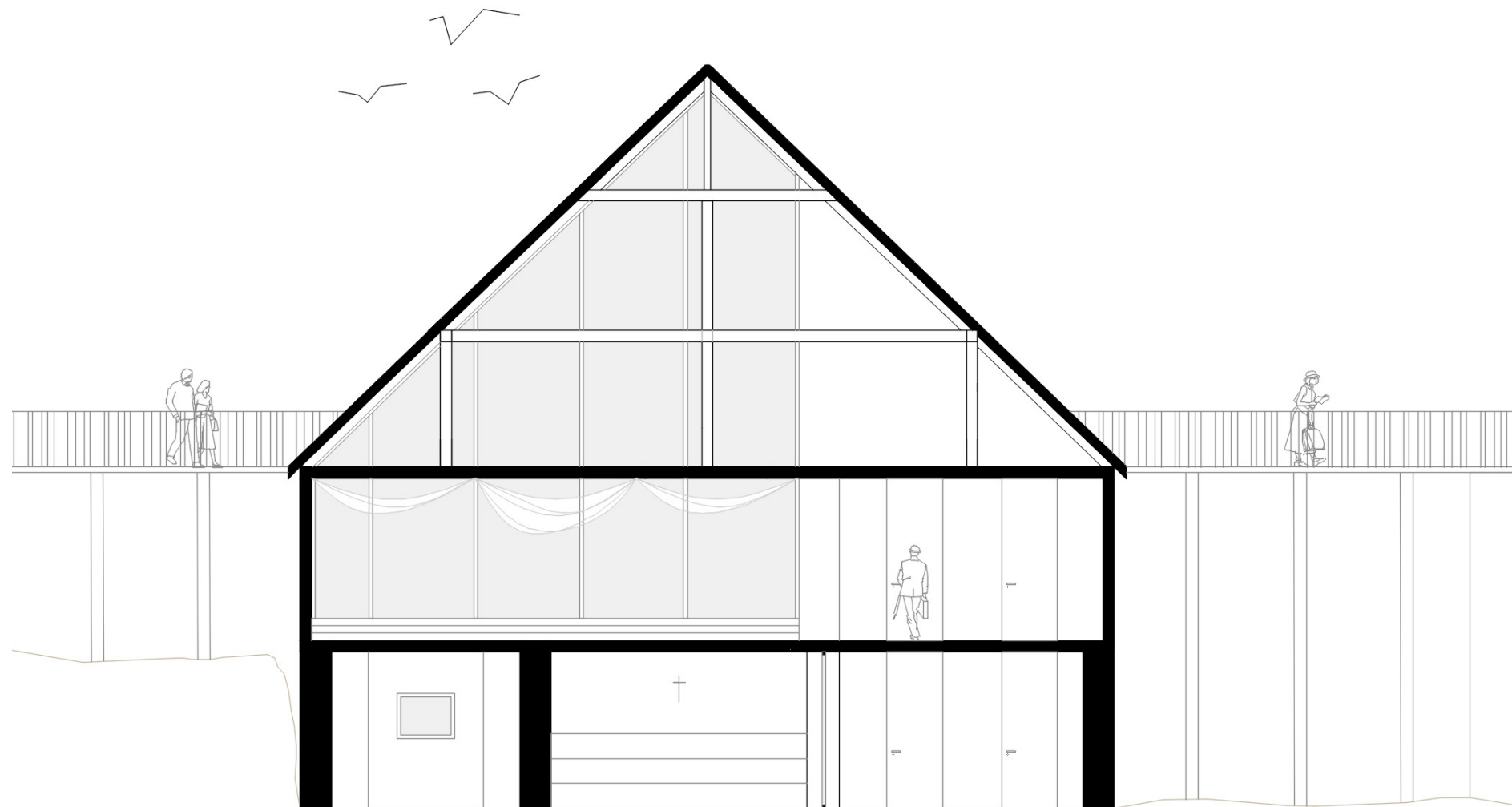
Schnitt M1:100
