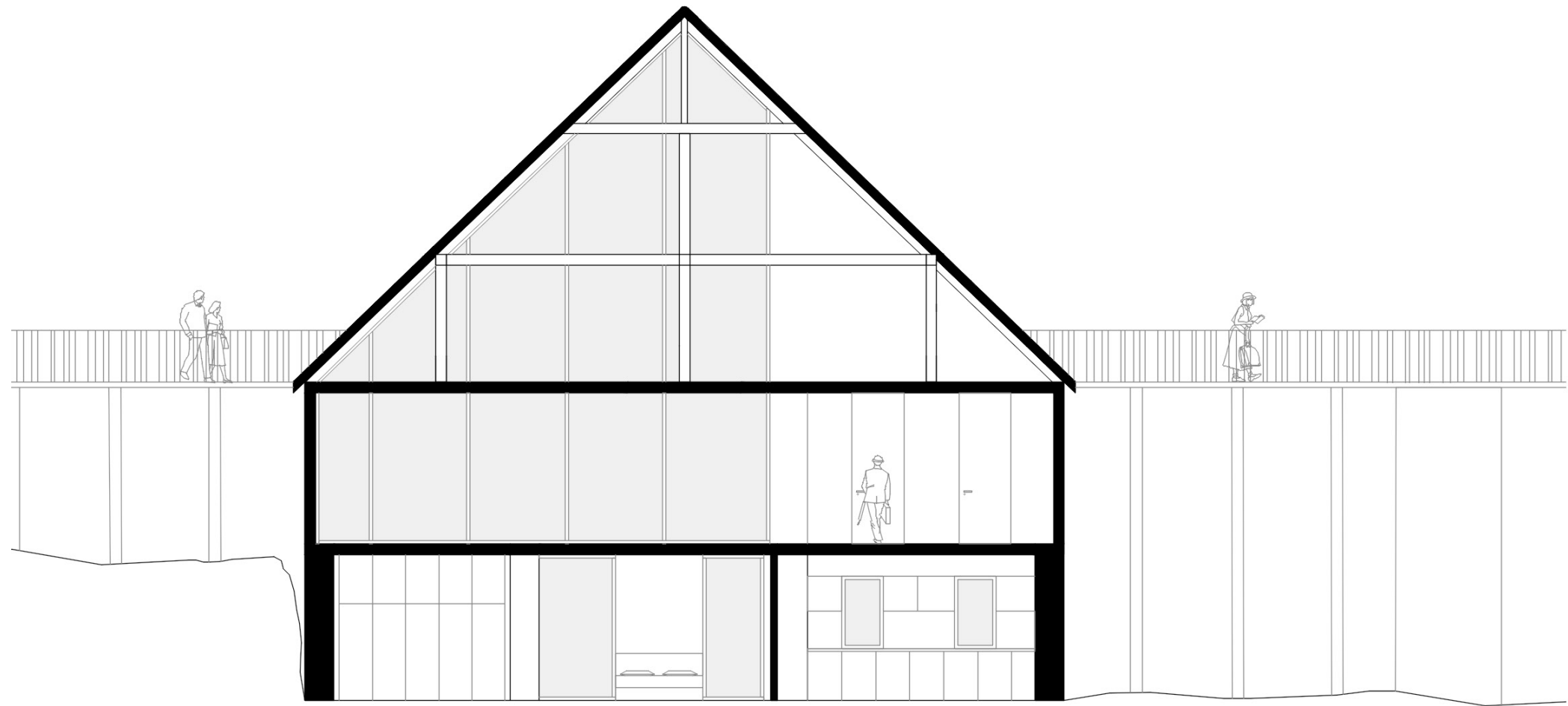
Schnitt M1:100
