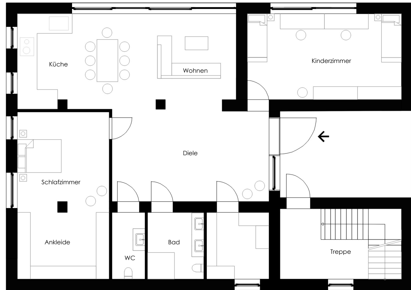
Erdgeschoss M1:100
