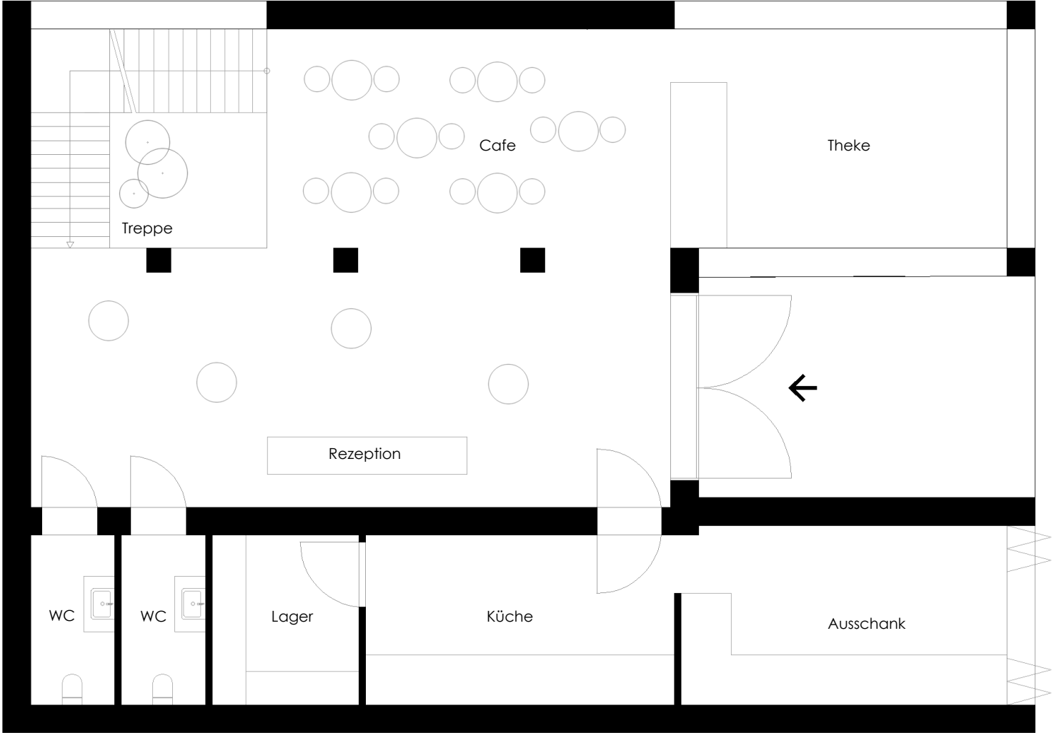
Erdgeschoss M1:100
