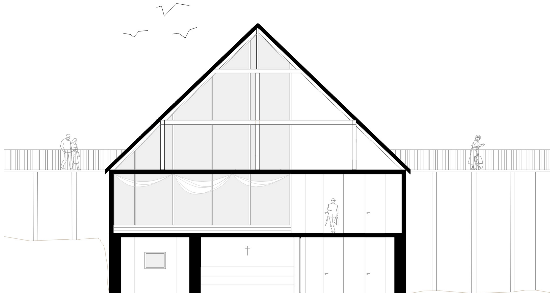
Schnitt M1:100
